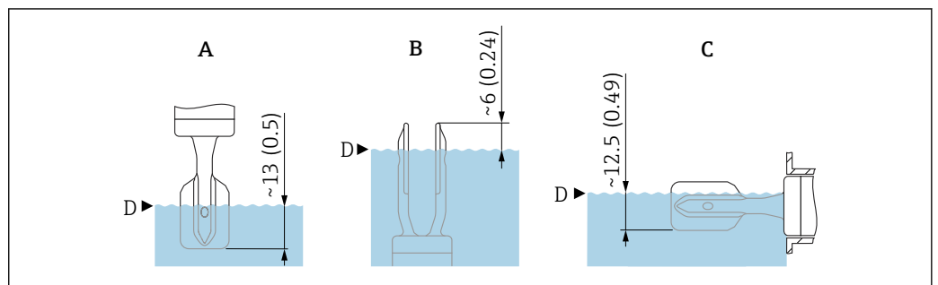
5 Puntos de conmutación típicos, diapason recubierto de plástico (ECTFE, PFA). Unidad de medida mm (in)
