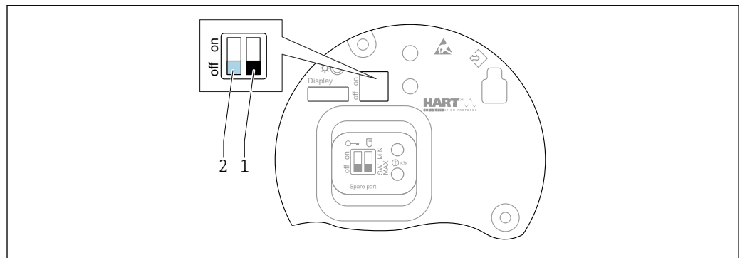
Fig. 28 Funciones de los microinterruptores en el módulo del sistema electrónico FEL60H
