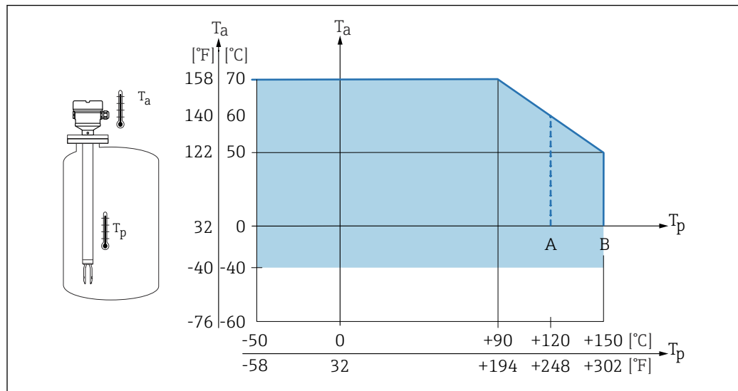
i 32 Temperatura ambiente admisible T_a en la caja en función de la temperatura de proceso T_p en el depósito
