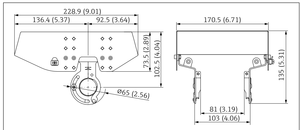
图 30 防护罩, 适用双腔体外壳。测量单位 mm (in)
