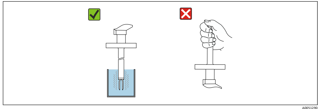
图 25 音叉的功能测试
