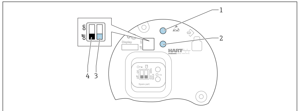
图 27 FEL60H 电子插件上的操作按键和 DIP 开关
