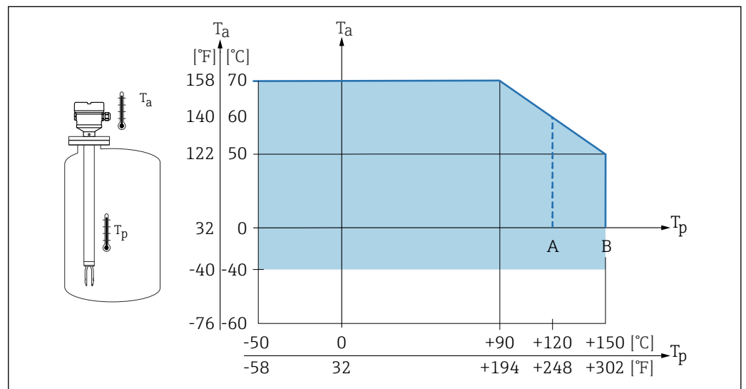
图 32 外壳允许环境温度 T_a 与罐体内部过程温度 T_p 的关系
