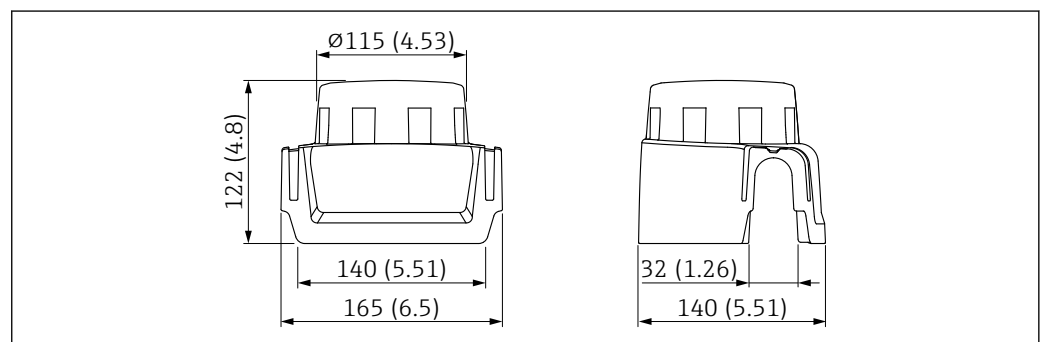
图 31 防护罩, 适用单腔体铝外壳。测量单位 mm (in)
