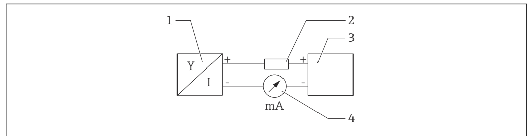
17 Блок-схема подключения HART
