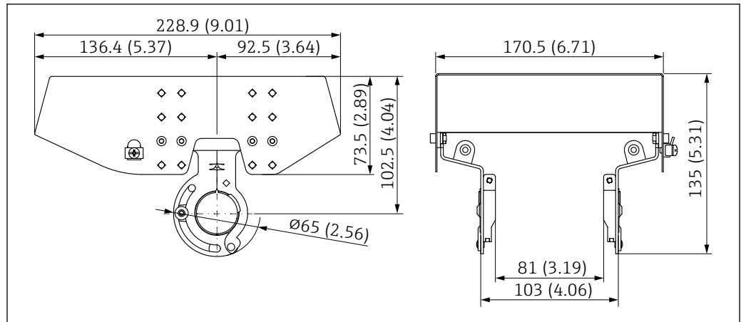
图 29 防护罩，适用双腔体外壳。测量单位 mm (in)
