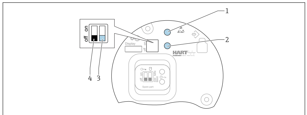
图 26 FEL60H 电子插件上的操作按键和 DIP 开关
