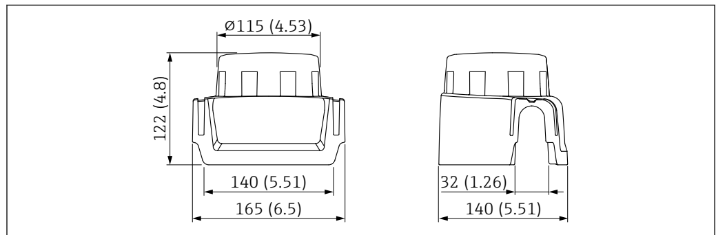
图 30 防护罩，适用单腔体铝外壳。测量单位 mm (in)
