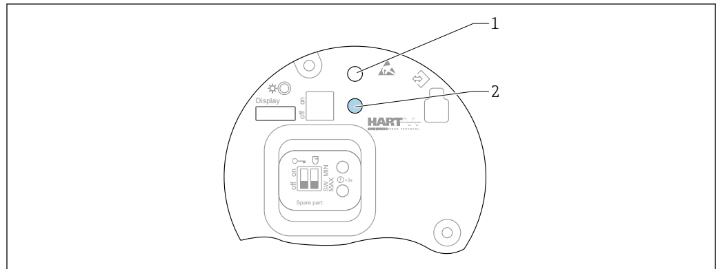
图 22 FEL60H 电子插件上的操作按钮
