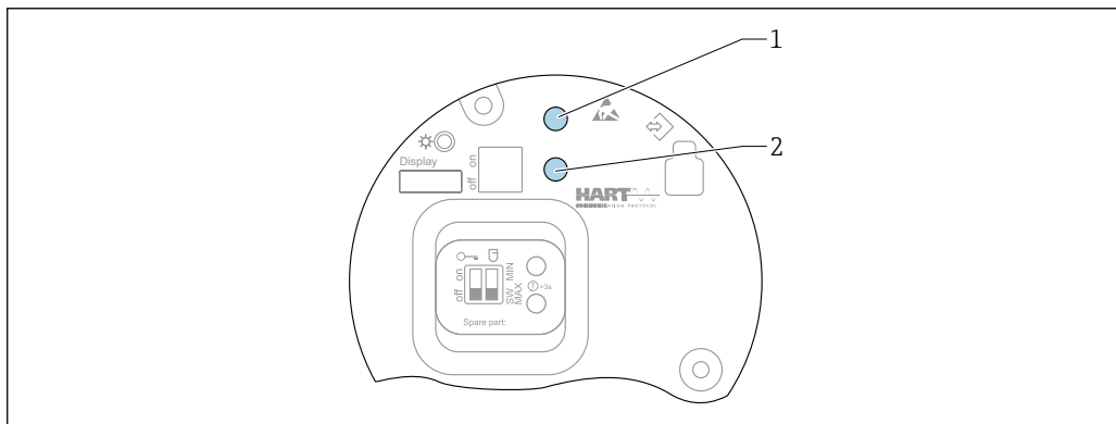
☑ 28 FEL60H 电子插件上的操作按键
