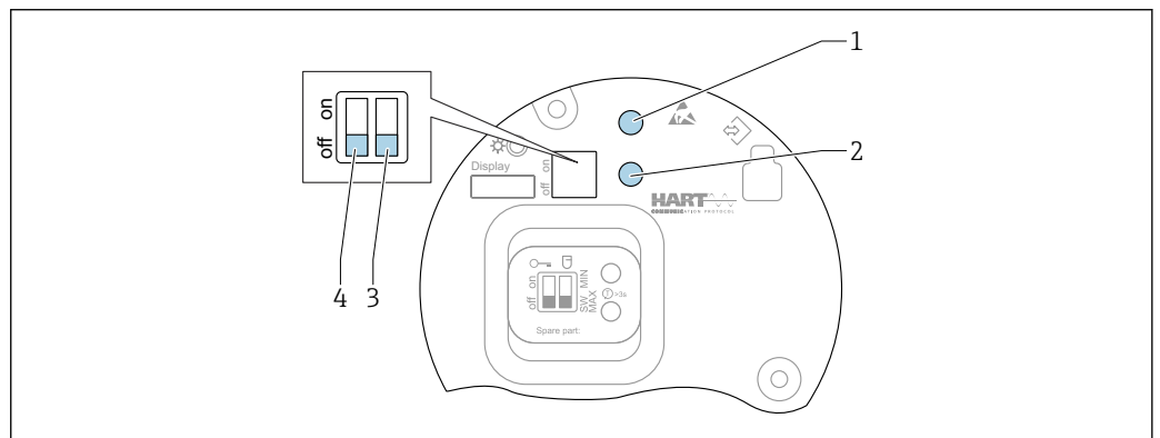
图 21 FEL60H 电子插件上的操作按键和 DIP 开关
