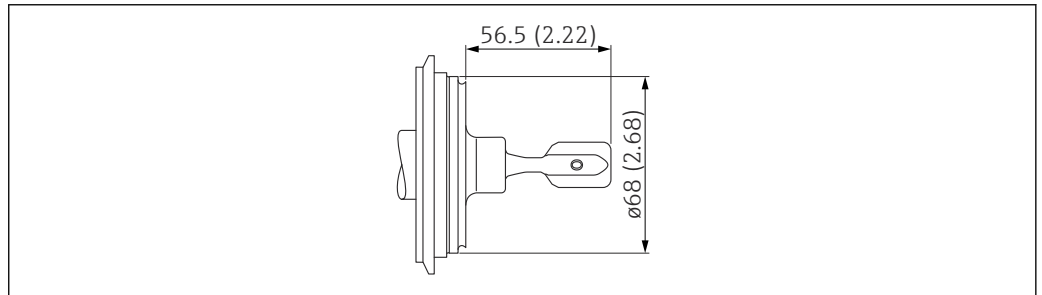
35 Varivent N 型接头, DN65-162 PN25 配合管道。测量单位 mm (in)
