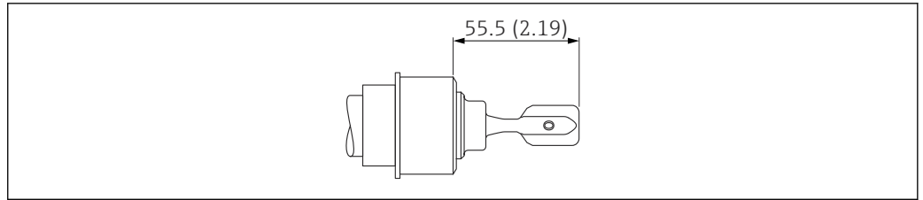
33 罐体接头（齐平安装在焊座中）。测量单位 mm (in)
