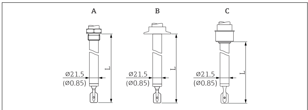
图 27 探头类型: 延长管型、短管型; (传感器长度 L)。测量单位 mm (in)
