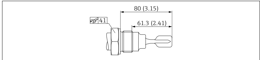
图 31 ISO228 G 1 螺纹。测量单位 mm (in)
