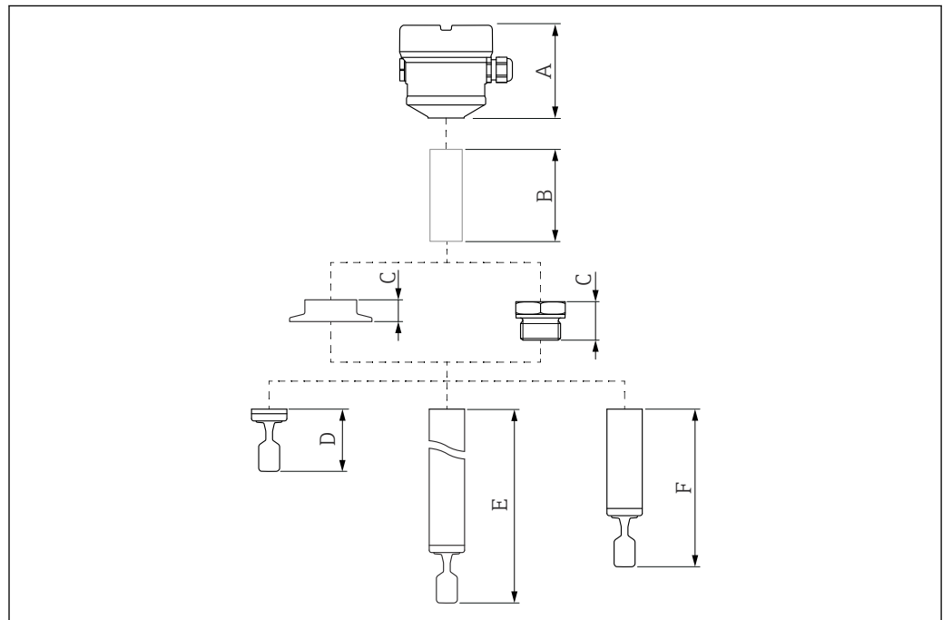
图 21 计算设备高度所需考虑的部件
