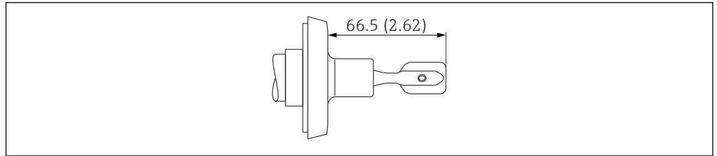
34 DIN11851 管接头。测量单位 mm (in)
