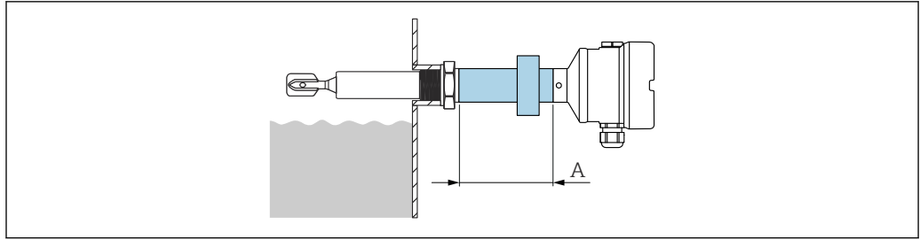
图 25 隔爆玻璃馈通 (搭配带延长管的仪表使用)
