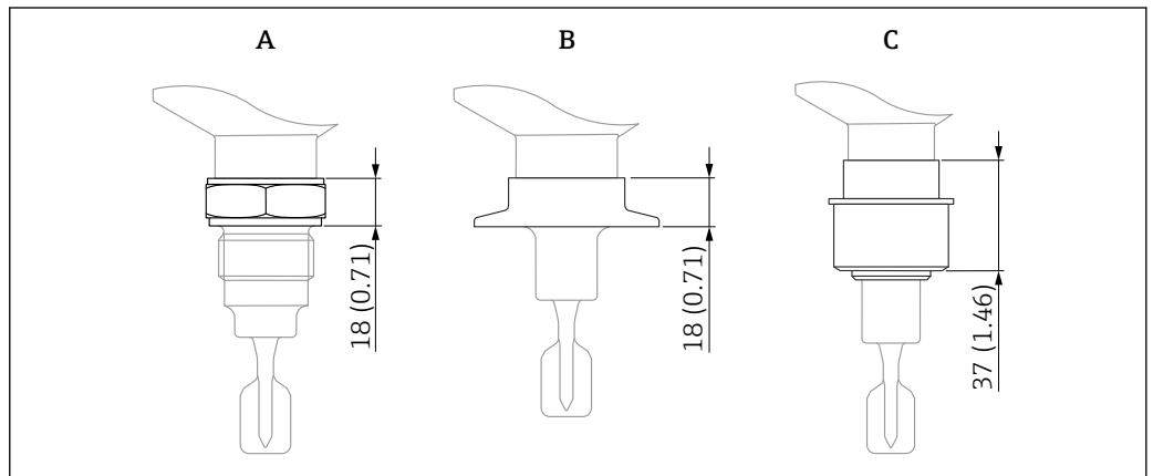
图 29 过程连接的最大高度规格。测量单位 mm (in)
