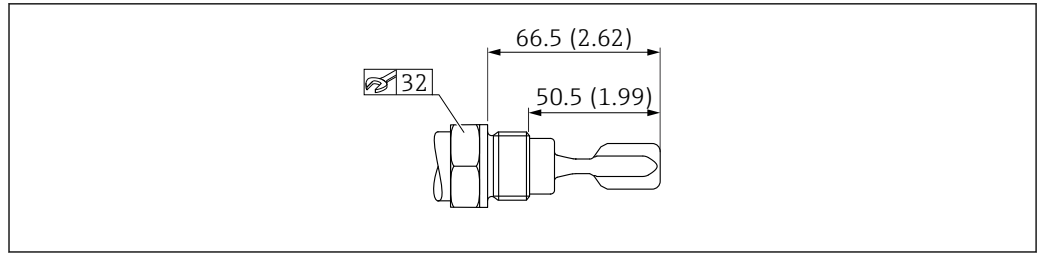
图 30 ISO228 G ¾ 螺纹。测量单位 mm (in)
