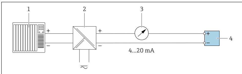
9 Przykład podłączenia wyjścia prądowego 4-20 mA (pasywnego)
