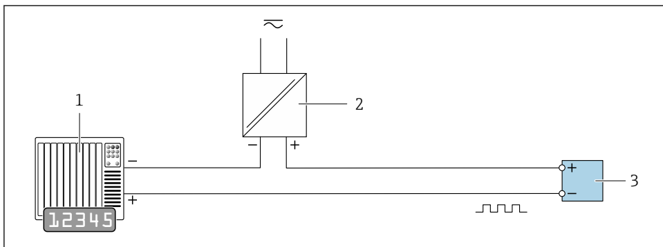
10 Przykład podłączenia wyjścia impulsowego/częstotliwościowego (pasywnego)
