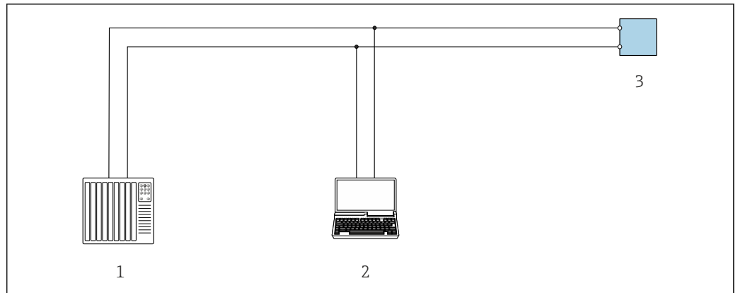
21 Opzioni per funzionamento a distanza mediante protocollo Modbus RS485 (attivo)
