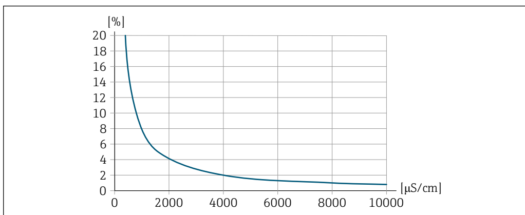
☰ 30 Ripetibilità in% del valore misurato - conducibilità elettrica [ \mu\text{S/cm} ]
