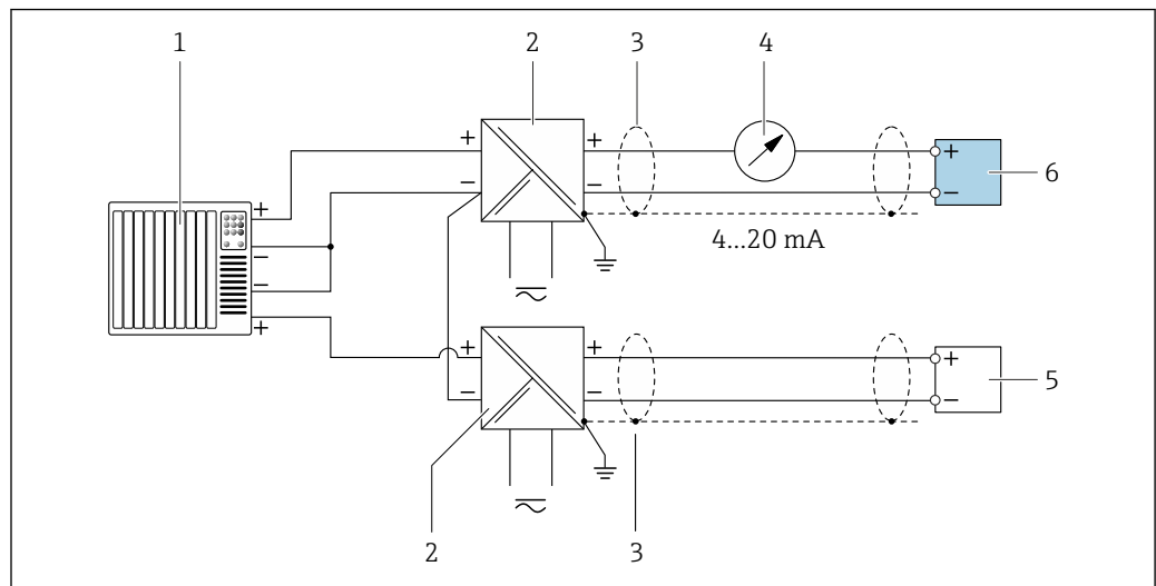
12 Esempio di connessione per ingresso HART con negativo comune (passivo)
