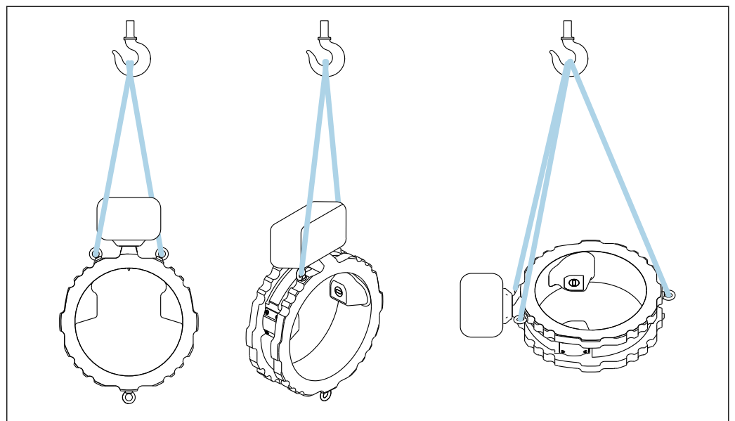
3 Trasporto verticale e orizzontale del dispositivo con ganci di sollevamento montati
