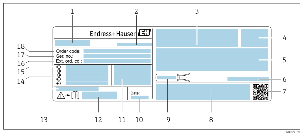
2 Esempio di targhetta trasmettitore
