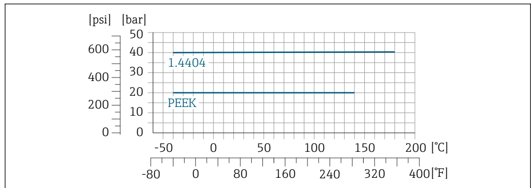
44 Con materiale giunto a compressione 1.4404/F316L/F316
