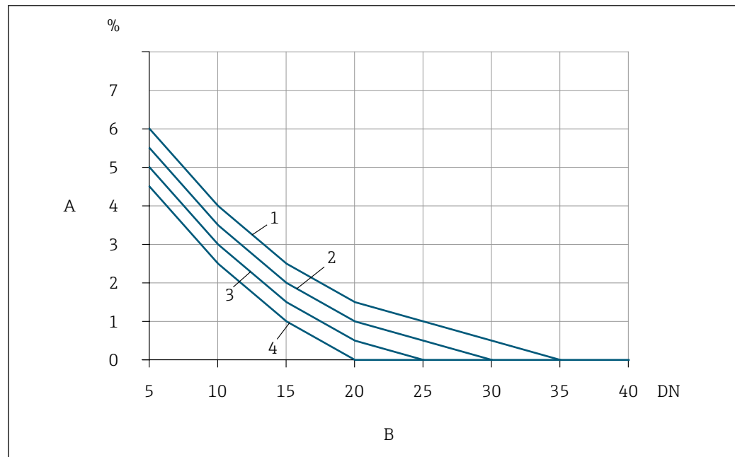
10 Errore di misura addizionale che ci si deve aspettare senza raddrizzatori di flusso a seconda del tipo di disturbo e del tratto in entrata
