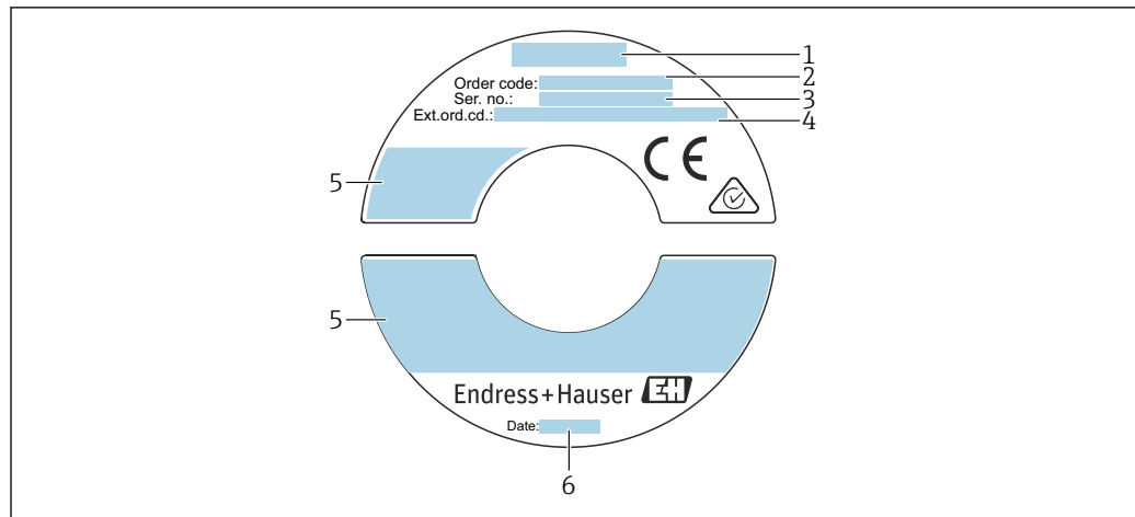
2 Esempio di targhetta del sensore
