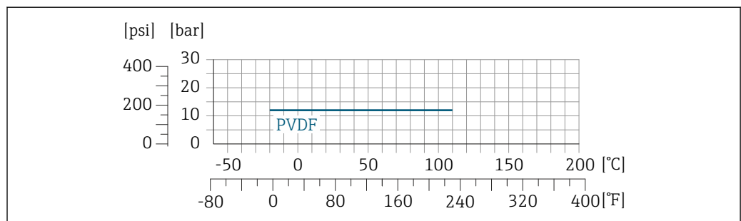
45 Con materiale giunto a compressione 1.4404/F316L/F316
