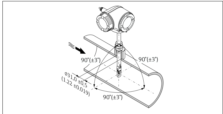
16 Unità ingegneristica: mm (in)
