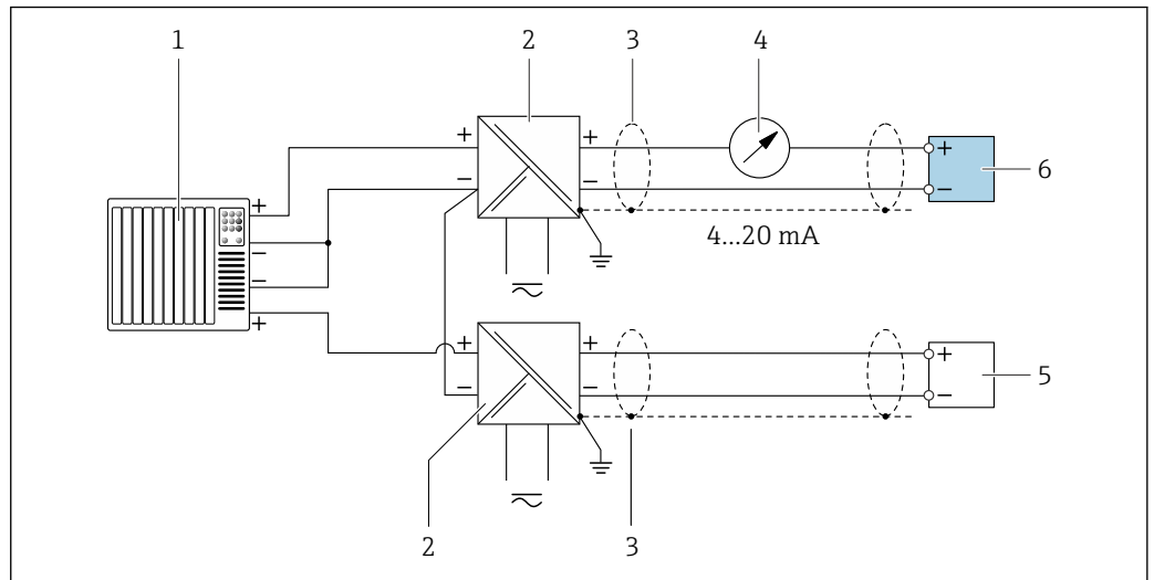
21 Esempio di connessione per ingresso HART con negativo comune (passivo)
