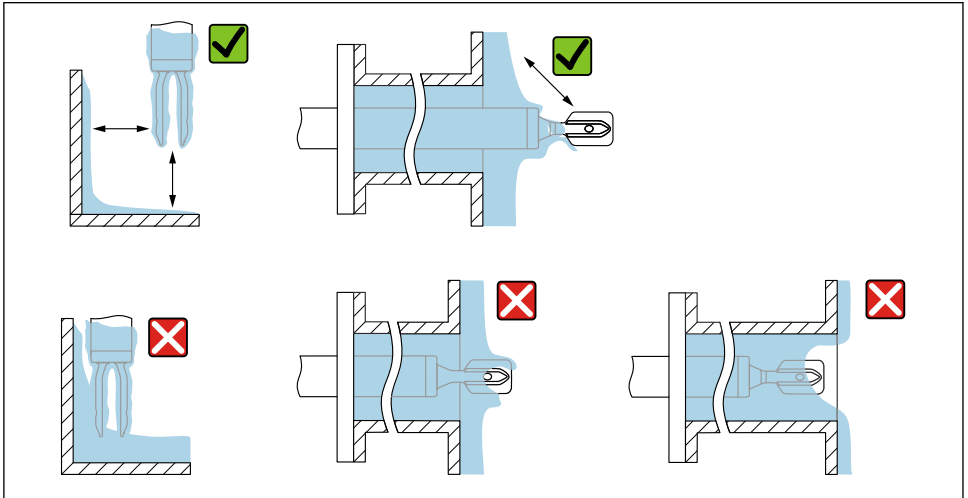
図 6 高粘度プロセス測定物の設置例
