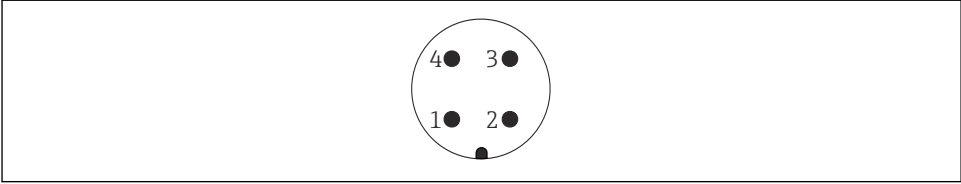
図 18 M12 プラグ、ピンの割当て
