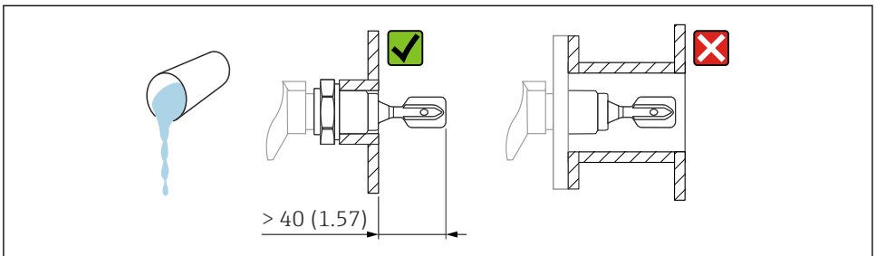
図 4 高粘度液体の設置例。測定単位 mm (in)
