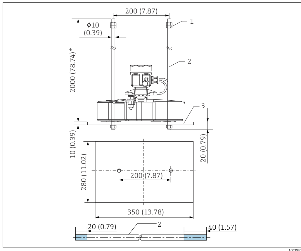
图 22 浮子导杆
