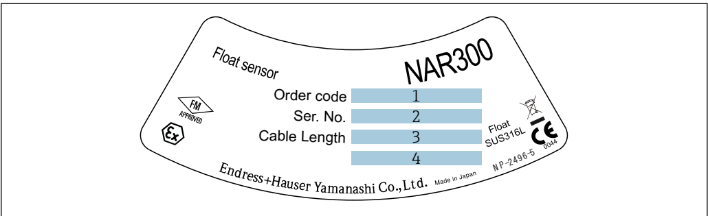
图 2 NAR300 铭牌
