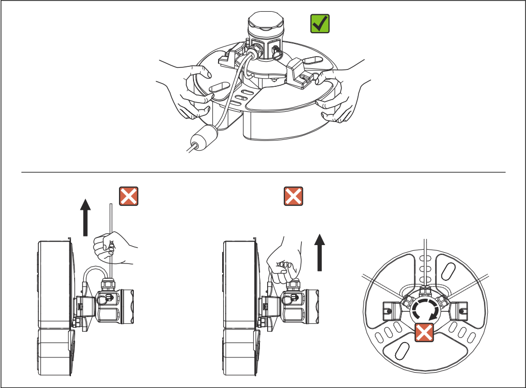
图 12 搬运 NAR300
