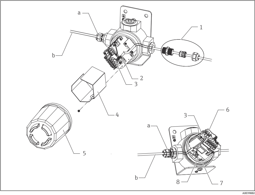
图 14 NAR300-x6xxxx 和防爆型传感器数据转换盒电缆安装示意图
