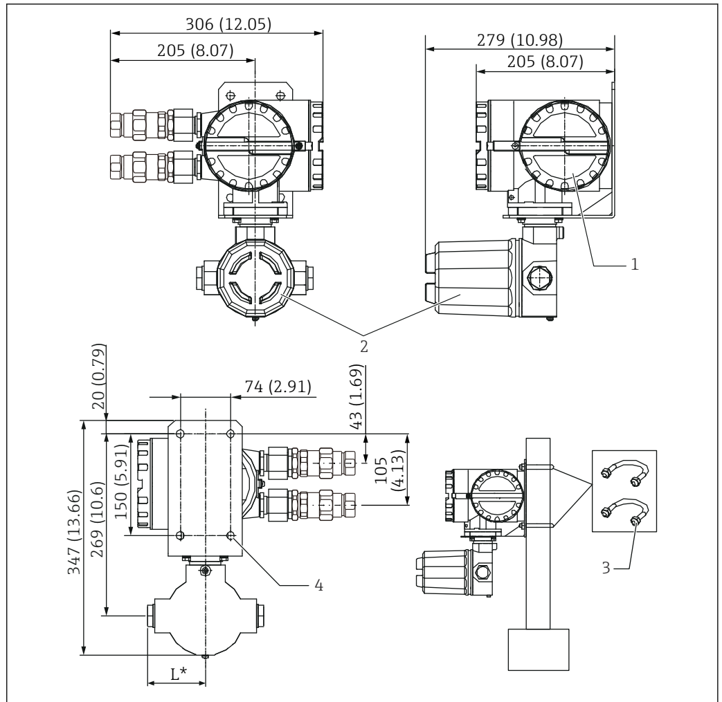
12 Encombrement du NRR261. Unité de mesure mm (in)
