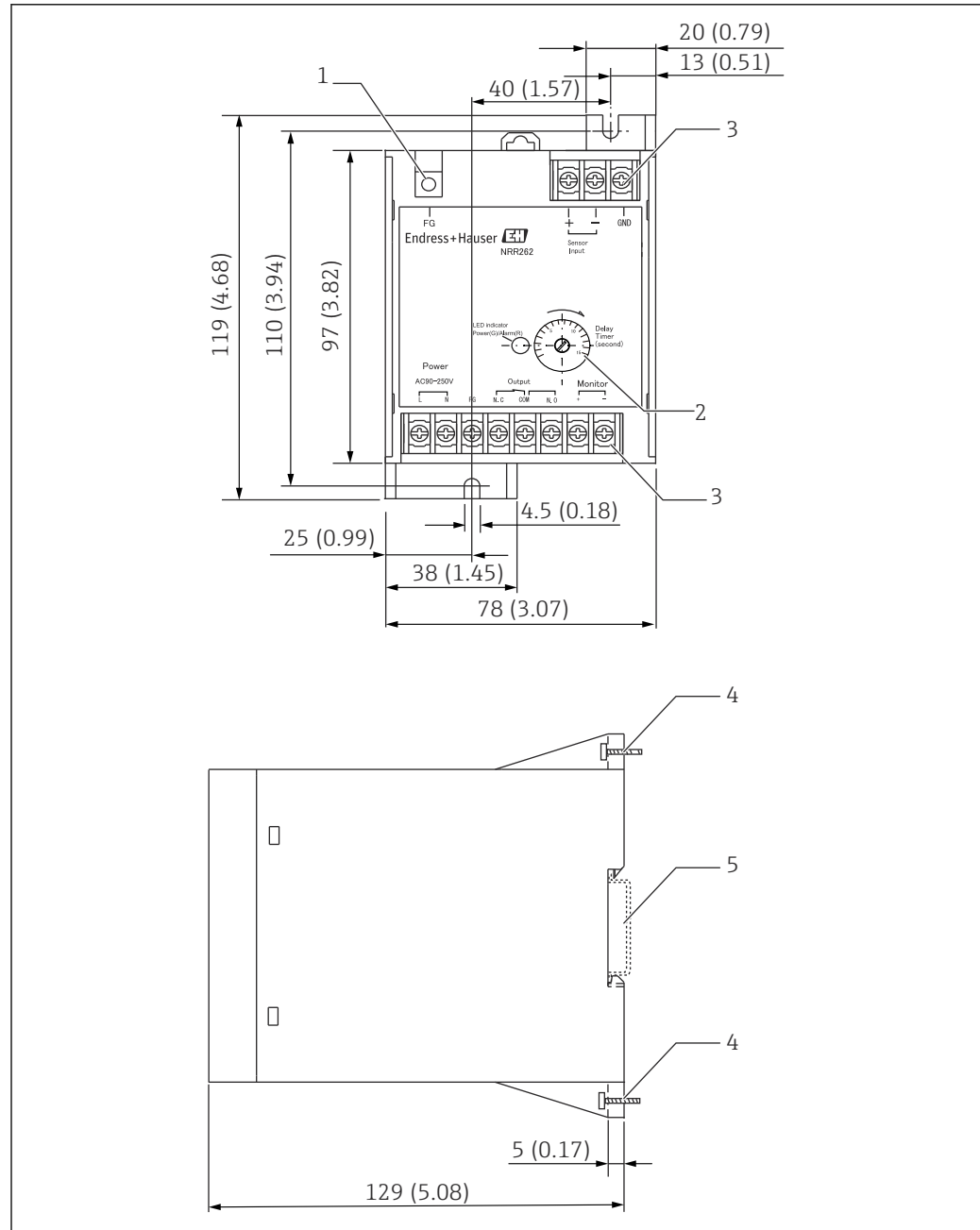
13 Encombrement du NRR262. Unité de mesure mm (in)
