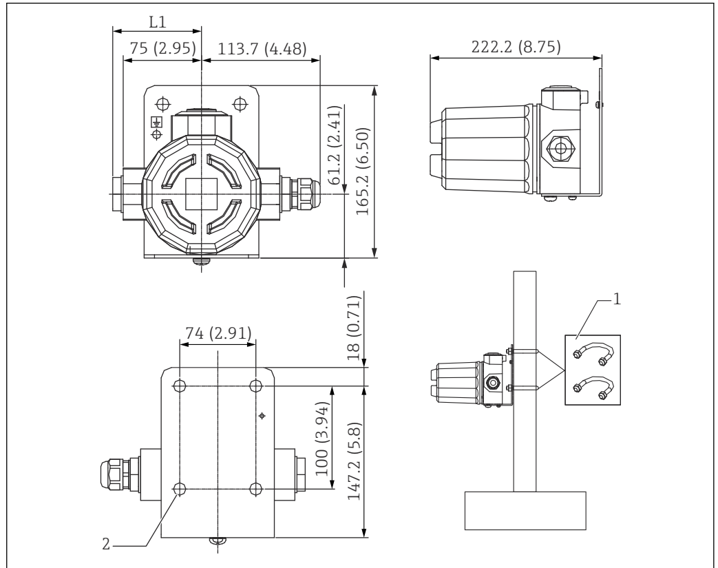
14 Encombrement du boîtier convertisseur Ex [ia]. Unité de mesure mm (in)
