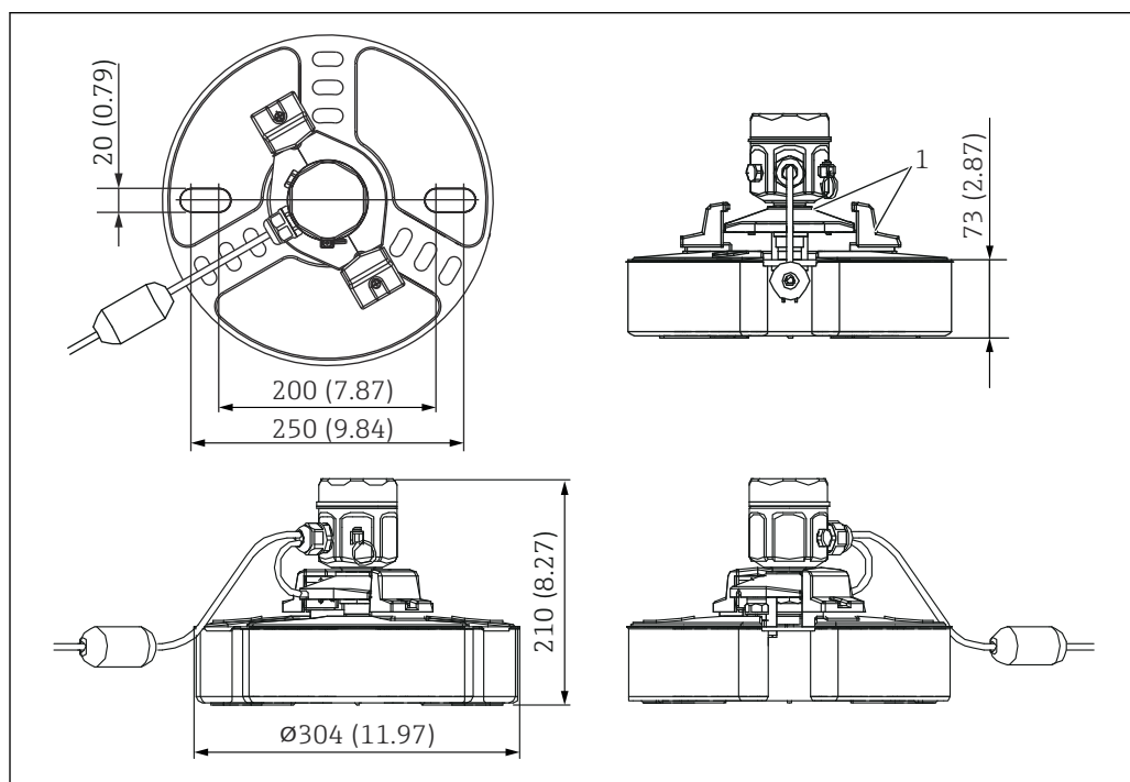
11 Внешний вид поплавкового датчика системы NAR300
