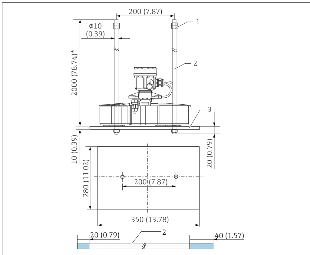
17 Направляющая поплавка
