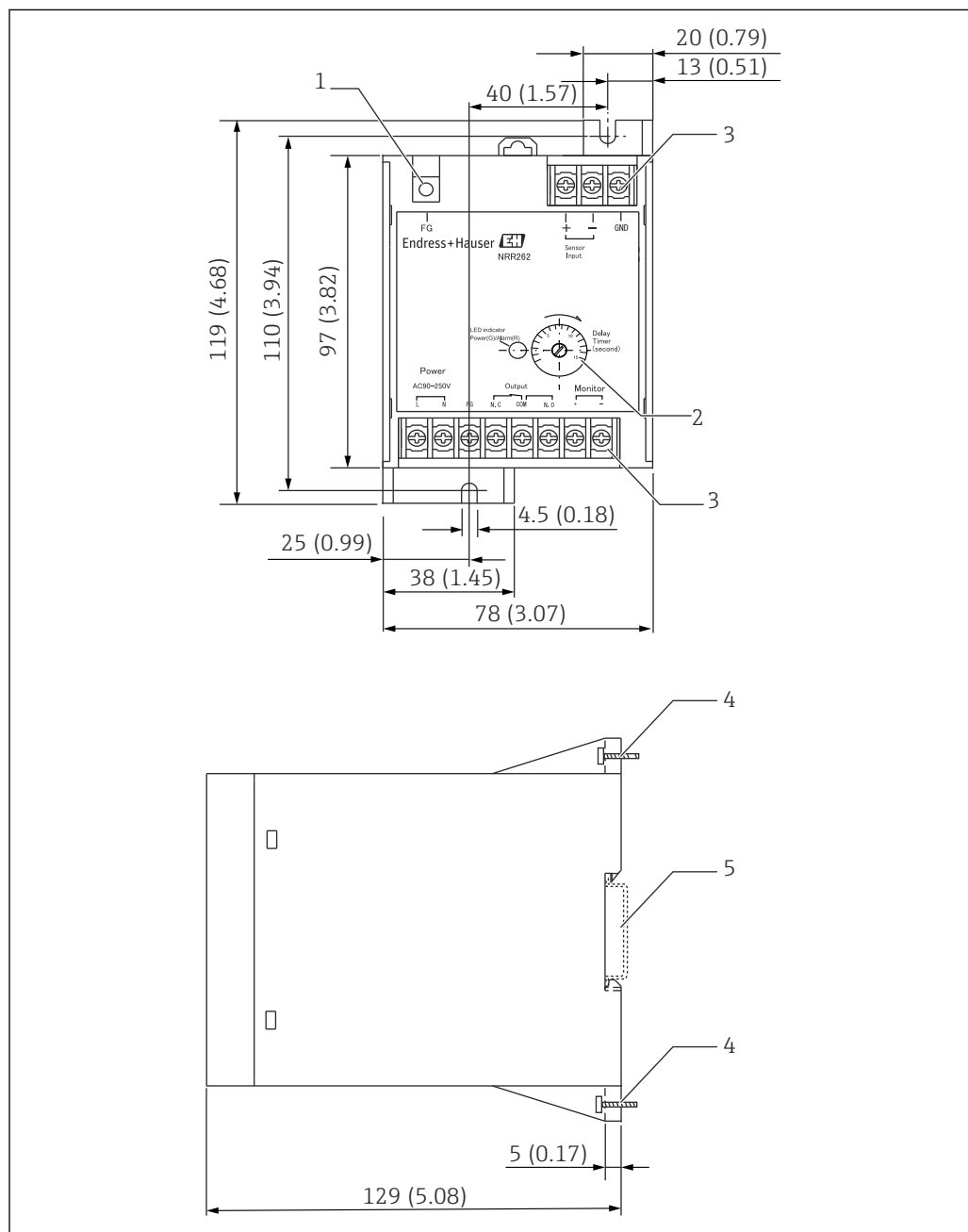
13 Внешний вид преобразователя NRR262. Единица измерения мм (дюйм)
