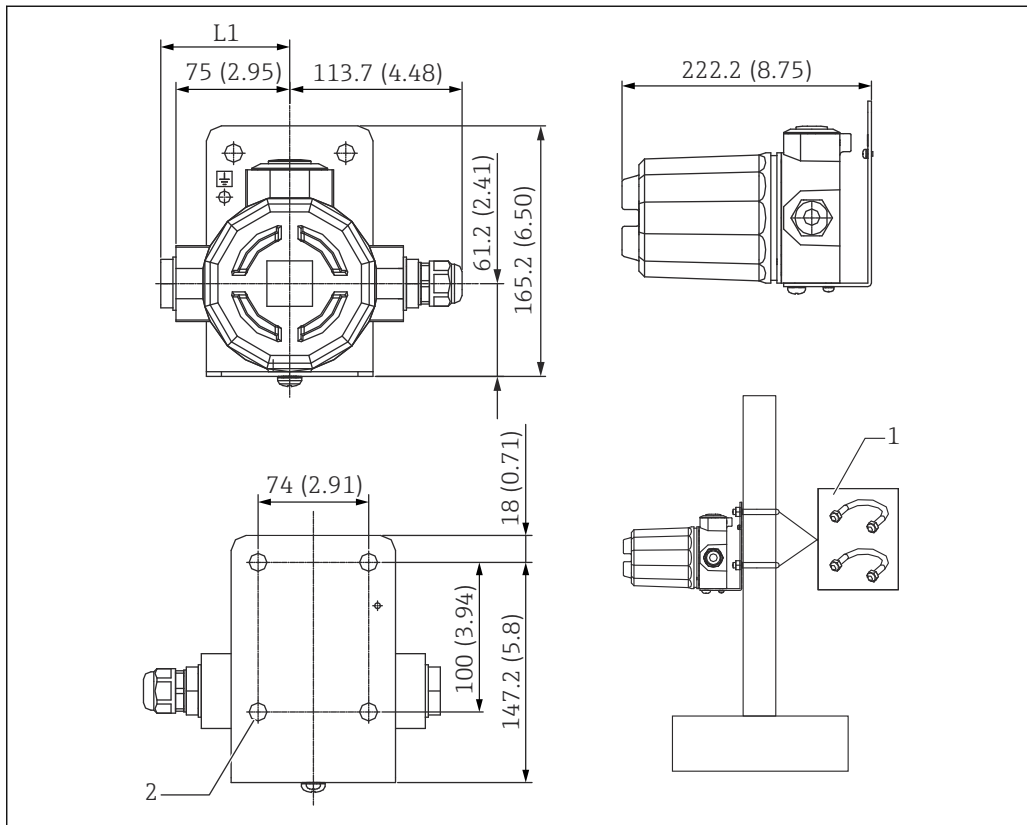
14 Внешний вид коробки датчика I/F Ex с взрывозащитой категории Ex [ia]. Единица измерения мм (дюйм)
