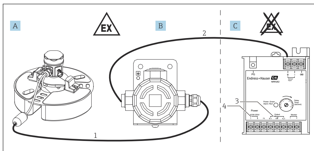
1 Вариант конфигурации системы 1
