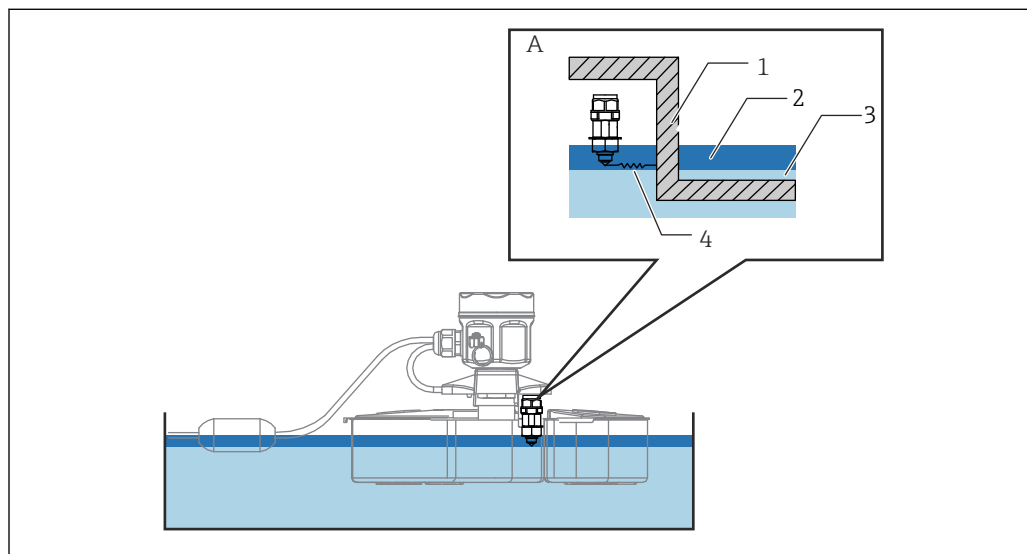
3 Принцип работы датчиков
