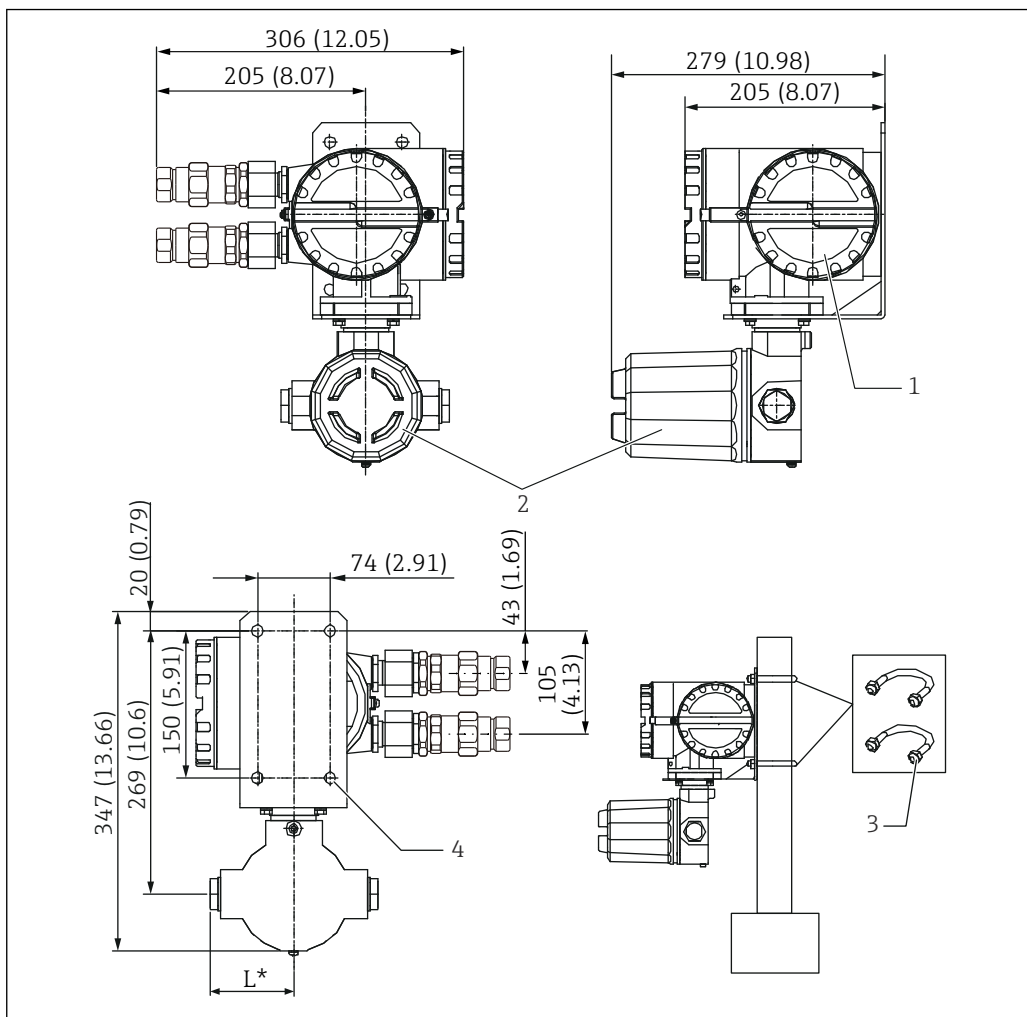
12 Внешний вид преобразователя NRR261. Единица измерения мм (дюйм)
