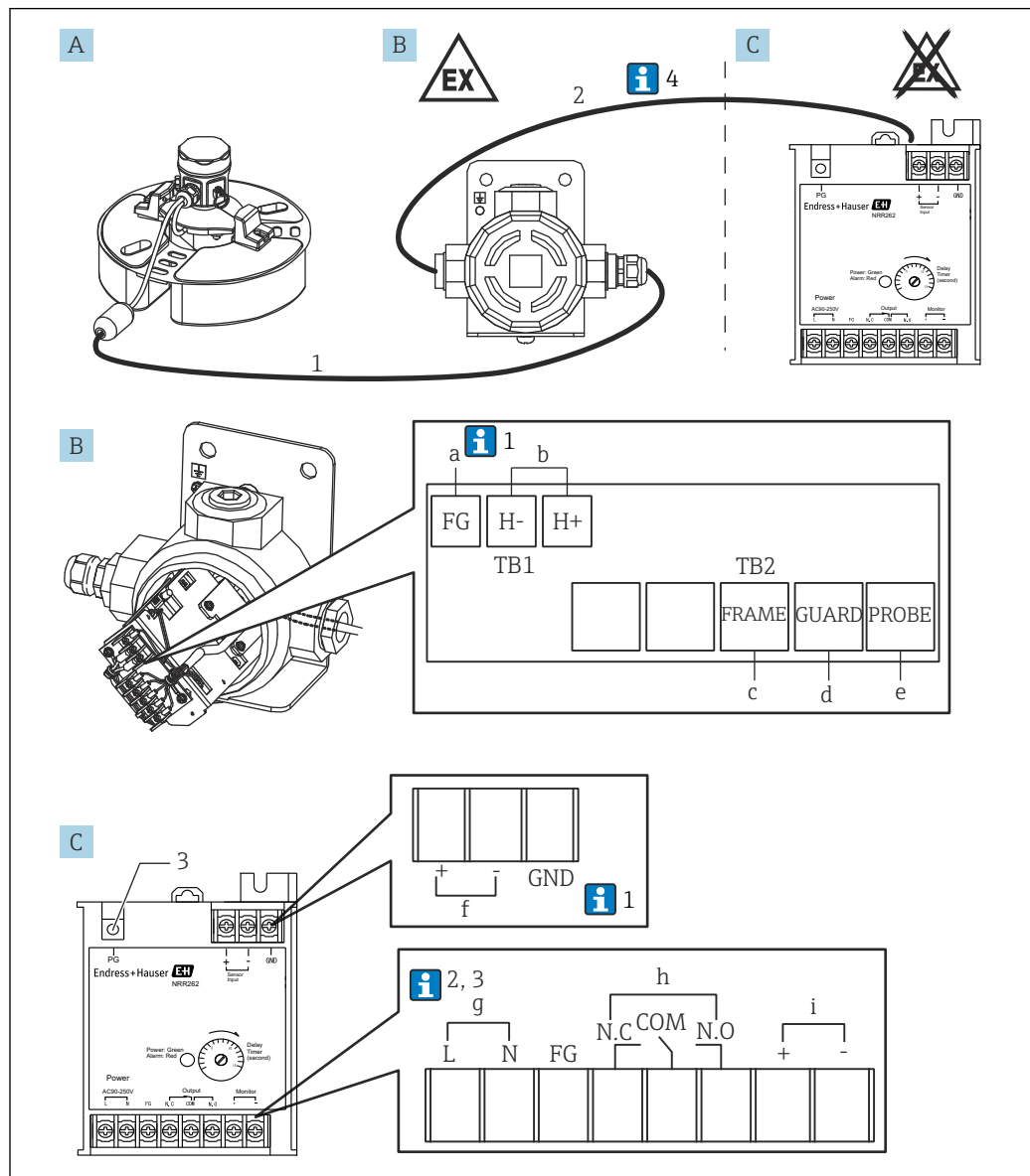
5 Подключение преобразователя Ex [ia] NRR262-4/A/B/C
