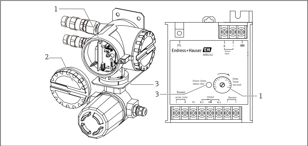
图 4 变送器 NRR261 (左) /变送器 NRR262 (右)
