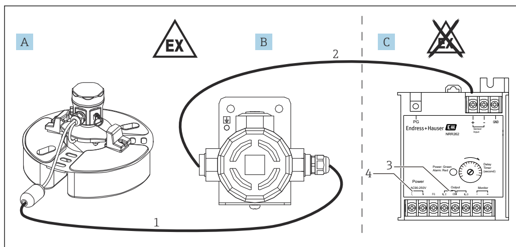
1 系统配置 1
