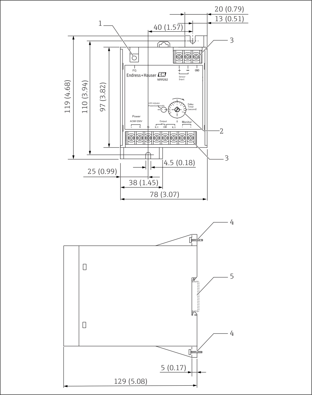
图 13 NRR262 的外形尺寸示意图。测量单位 mm (in)
