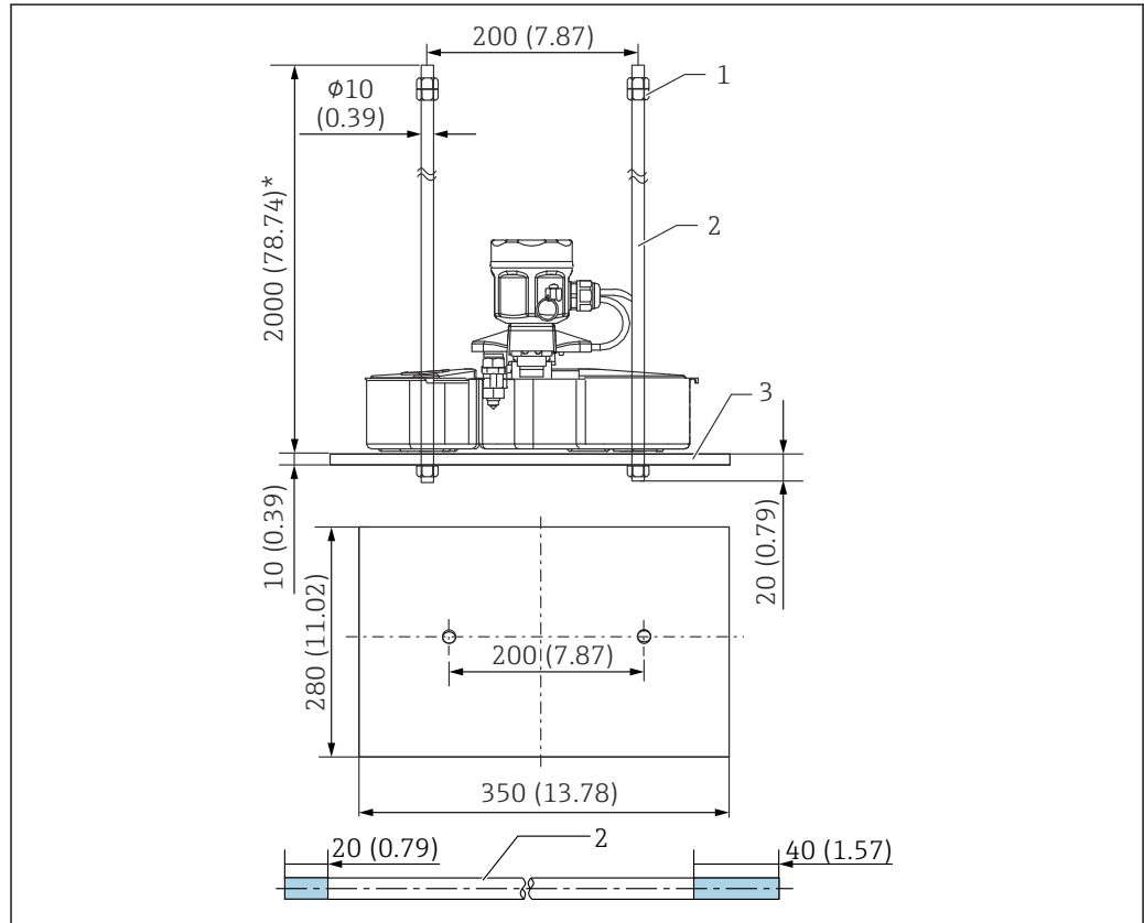
图 10 NAR300, 浮子导杆
