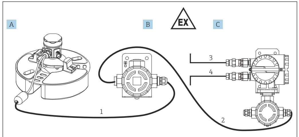
图 2 系统配置 2
