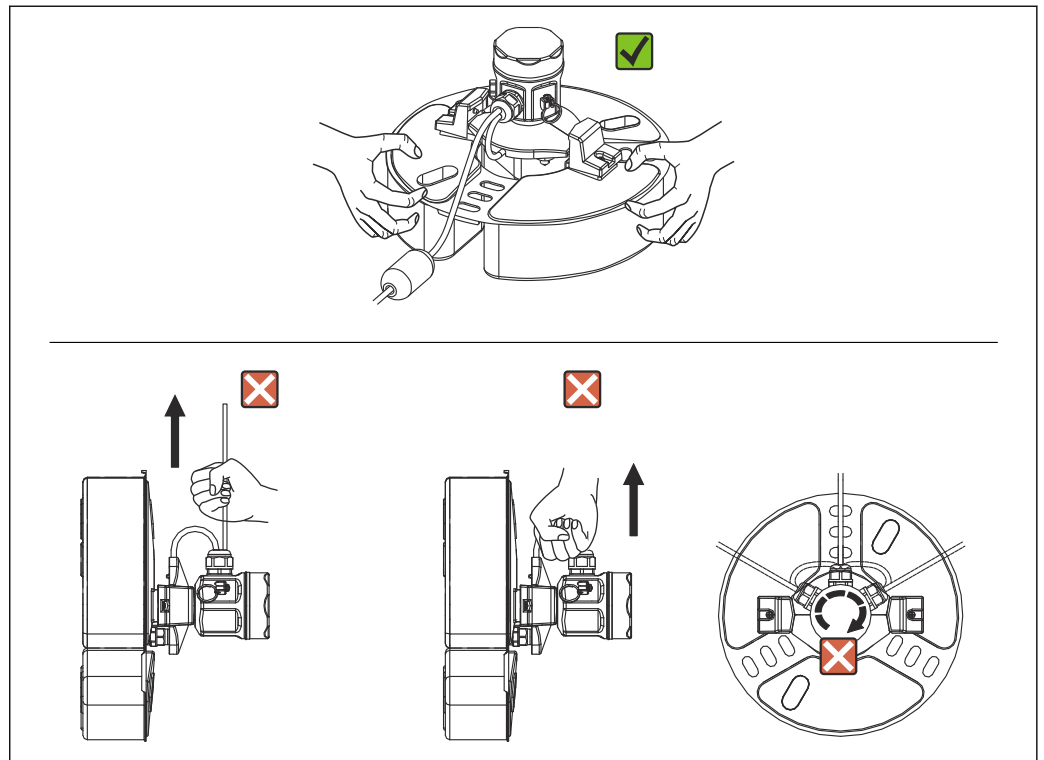
图 9 搬运 NAR300
