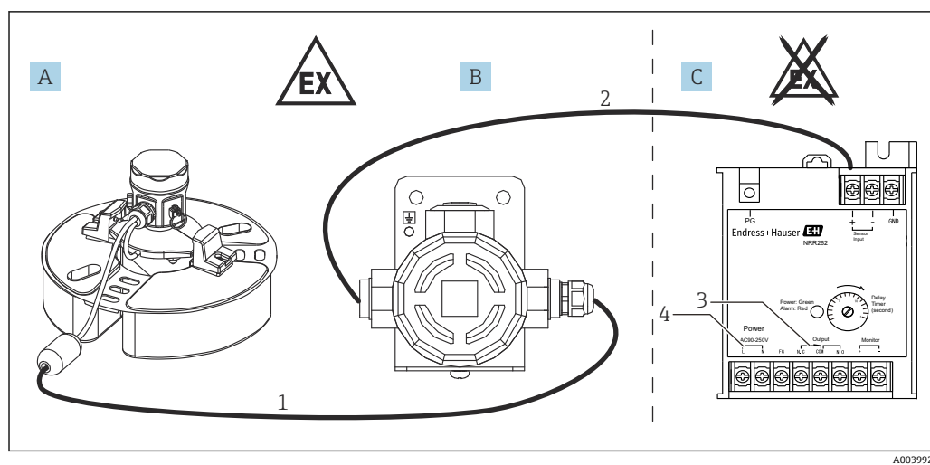
图 15 系统配置 1
