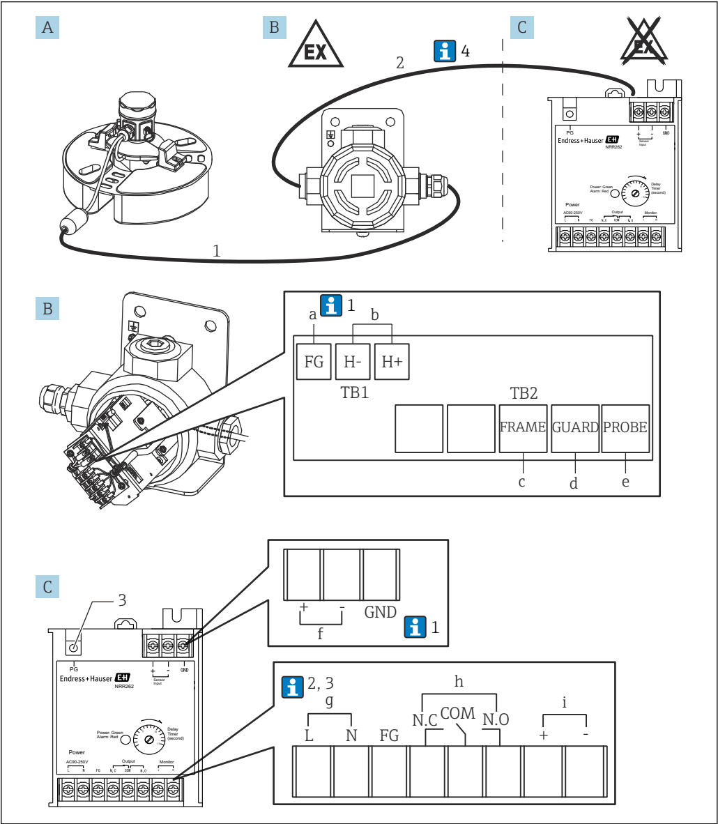
图 5 本安防爆型 (Ex [ia]) 转换器 NRR262-4/A/B/C 接线示意图
