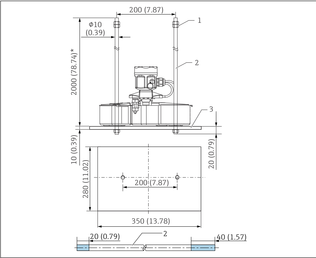
图 17 浮子导杆 1 螺母 (M10) 2 浮子导杆 3 重量
