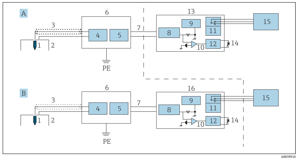
图 7 接线图
