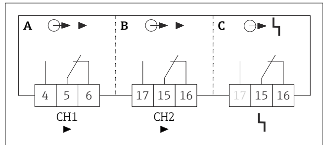
4 Conectarea ieșirilor
