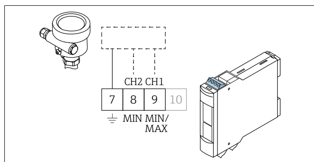
2 Conexão de aterramento de proteção, MIN e MAX dependendo do sensor, consultar o manual do sensor
