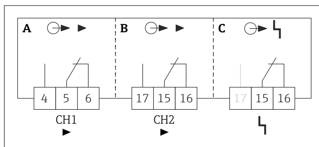
4 Raccordement des sorties
