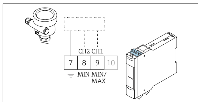
2 Raccordement de la terre de protection, MIN et MAX en fonction du capteur, voir le manuel du capteur
