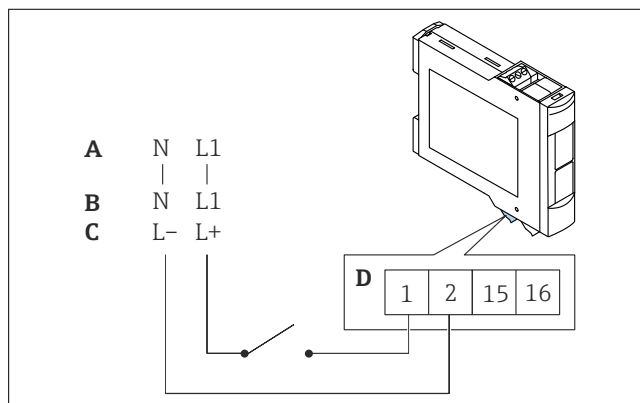
3 Rozmieszczenie zacisków
