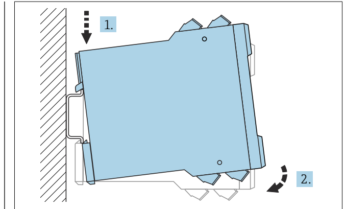
1 Montaj; EN 60715 TH35-7.5/EN 60715 TH35-15'e göre DIN ray
