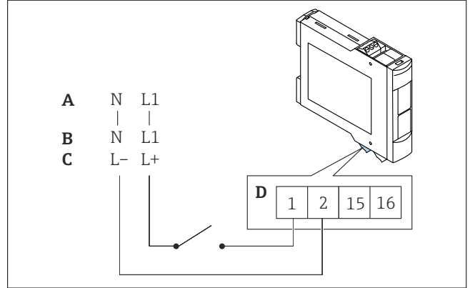
3 Terminal düzenlemesi
