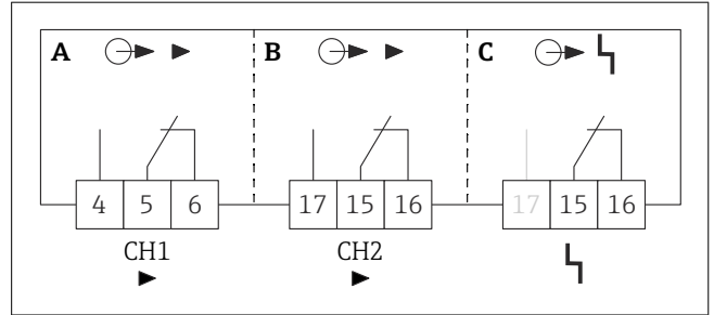
4 Çıkışların bağlanması
