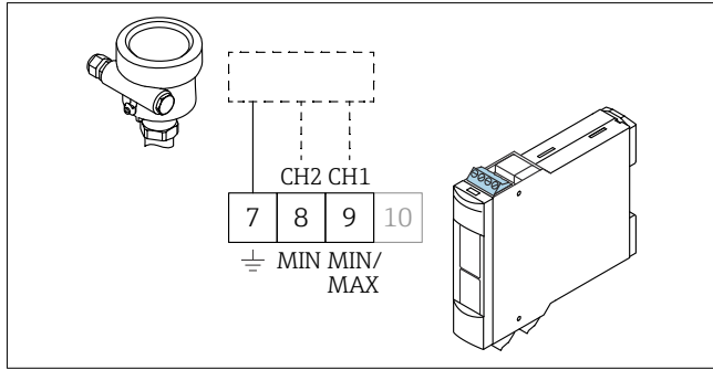
2 Korumucu topraklama bağlantısı, MIN ve MAX sensöre bağlıdır, sensör kılavuzuna bakın
