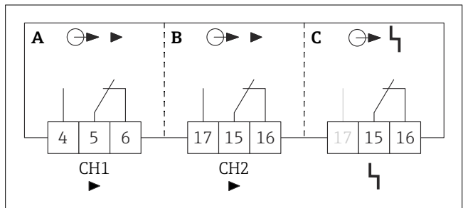
4 Подключение выходов
