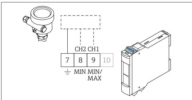
2 Подключение защитного заземления, минимальный уровень (MIN) и максимальный уровень (MAX) в зависимости от датчика, см. руководство по эксплуатации датчика
