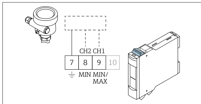
2 Anschluss von Schutzleiter, MIN und MAX abhängig vom Messaufnehmer, siehe Anleitung vom Messaufnehmer
