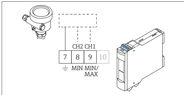
図2 保護接地接続 (下限 (MIN) と上限 (MAX) はセンサに応じて異なります。センサのマニュアルを参照)
