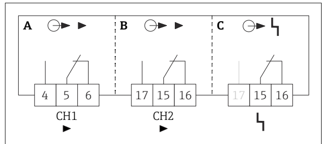
図4 出力の接続
