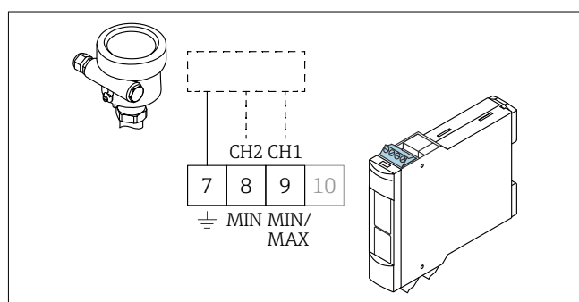
2 Beskyttende jordforbindelse, MIN og MAX avhengig av sensoren, se sensorens bruksanvisning
