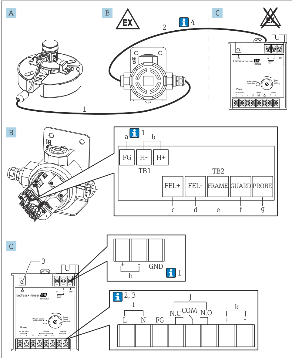
15 Câblage du convertisseur Ex [ia] NRR262-4/A/B/C
