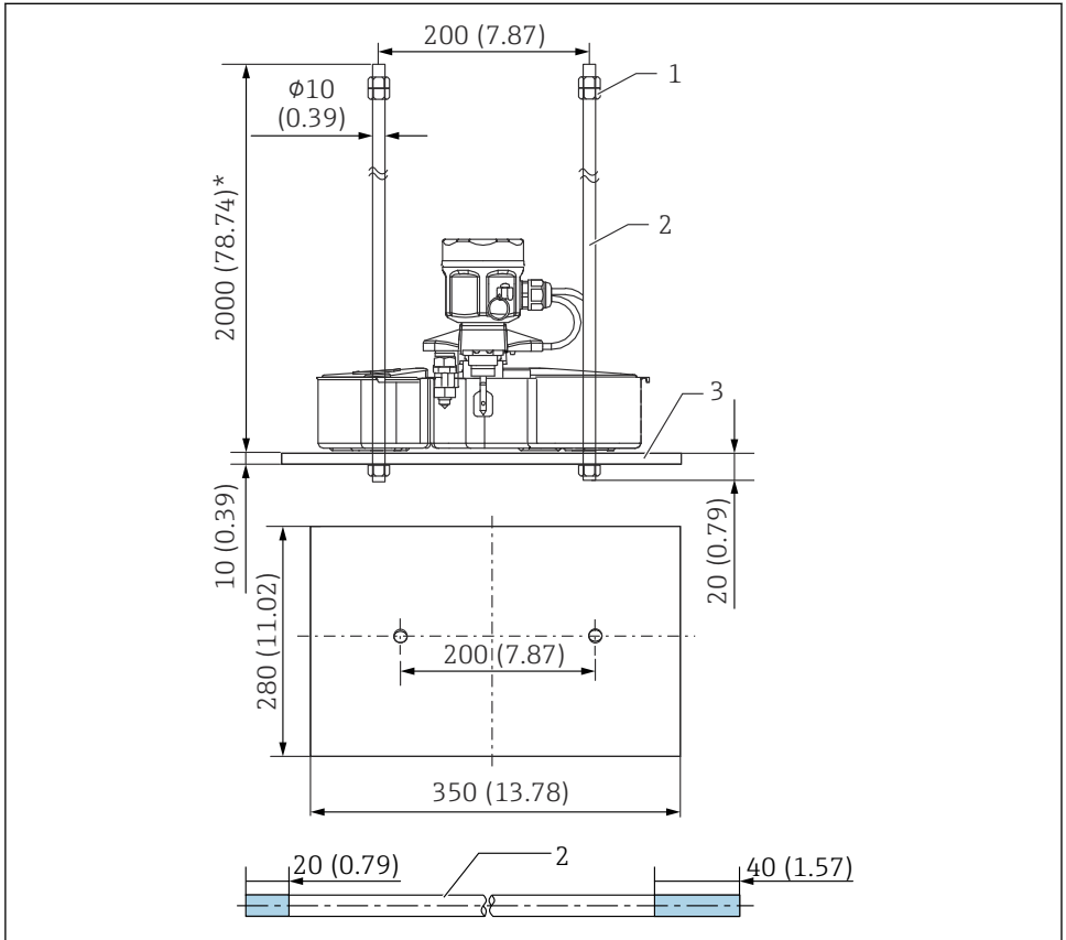
9 NAR300, guide de flotteur. Unité de mesure mm (in)
