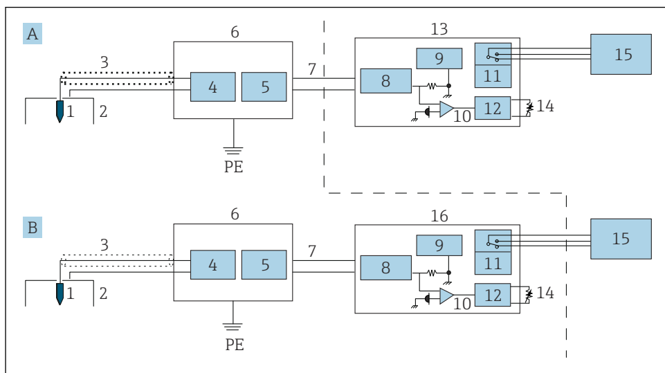
14 Schemat połączeń
