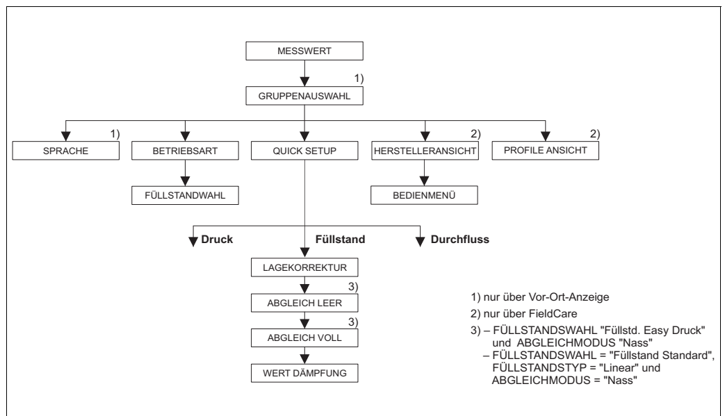
Abb. 32: Quick Setup-Menü für die Betriebsart "Füllstand"
