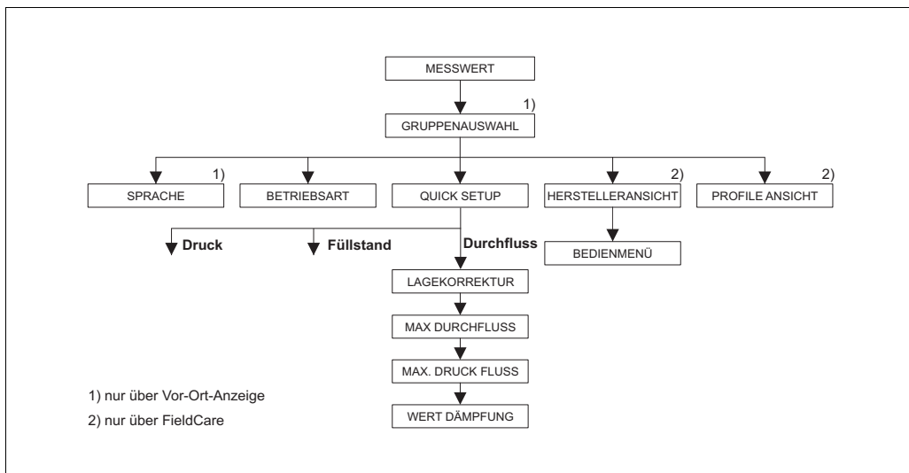
Abb. 28: Quick Setup-Menü für die Betriebsart "Durchfluss"
