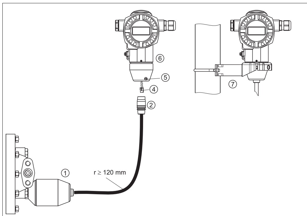
Abb. 16: Variante "abgesetztes Gehäuse"
