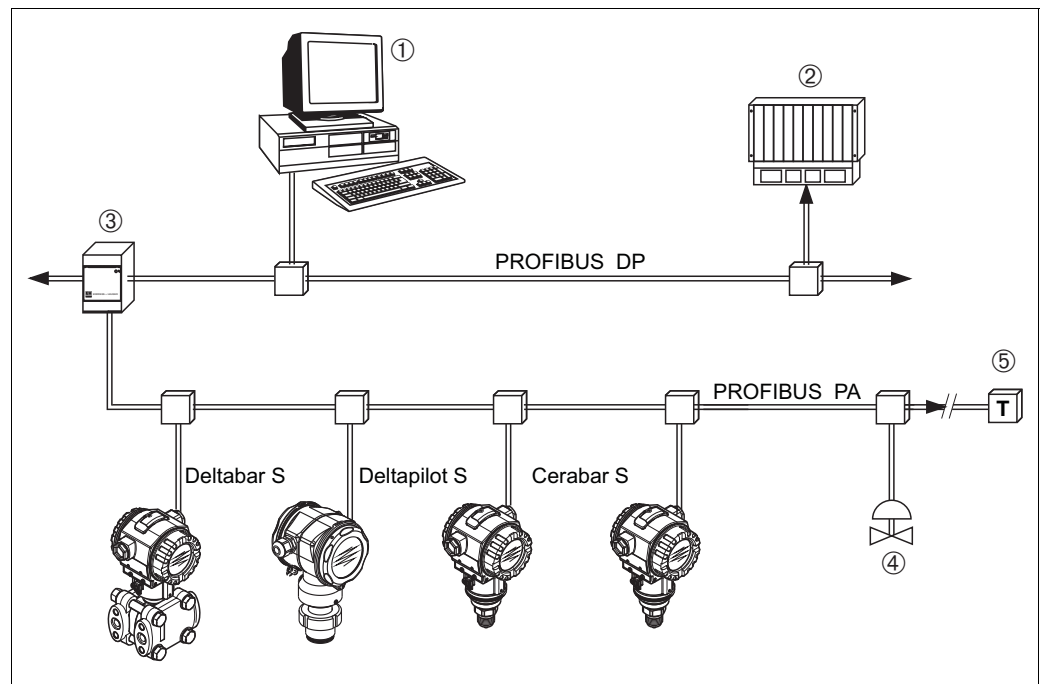
Abb. 21: Systemarchitektur PROFIBUS
