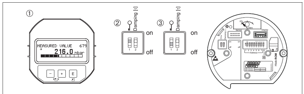
Abb. 26: Lage DIP-Schalter "Hardware-Verriegelung" auf dem Elektronikensatz
