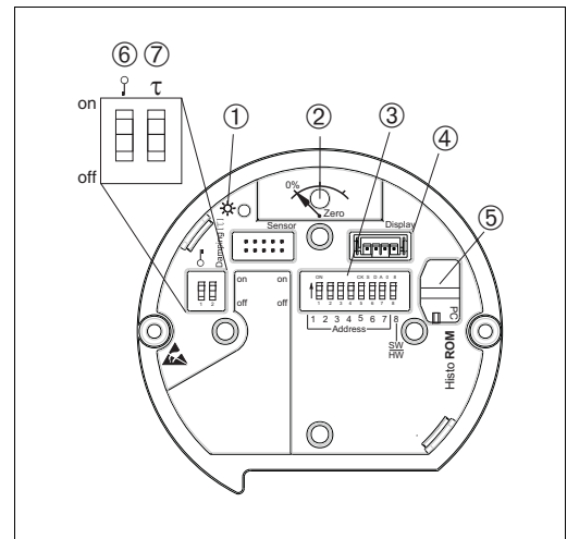
Abb. 20: Bedientaste und Bedienelemente innen
