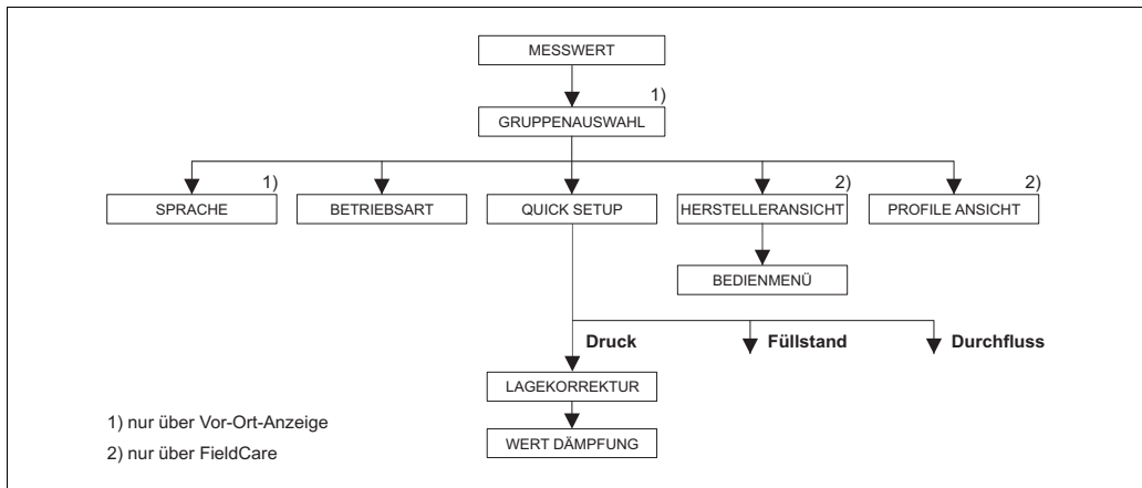
Abb. 34: Quick Setup-Menü für die Betriebsart "Druck"
