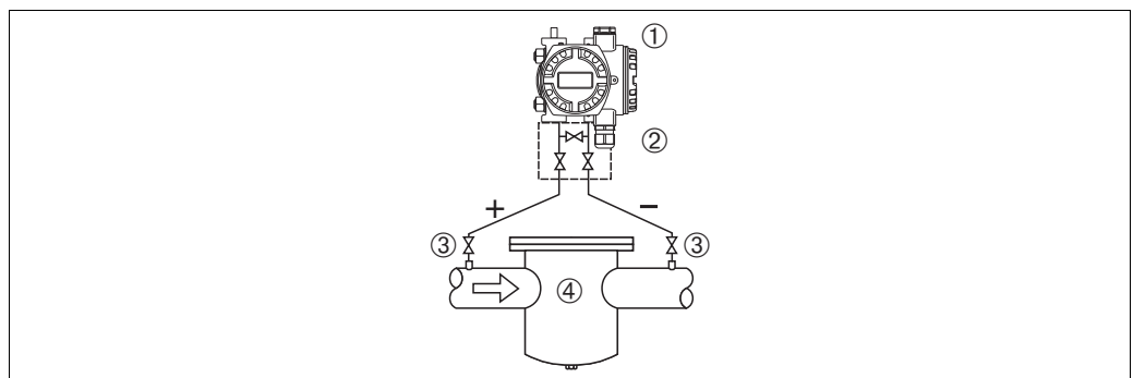
Abb. 11: Messanordnung Differenzdruckmessung in Gasen und Dämpfen mit PMD75
