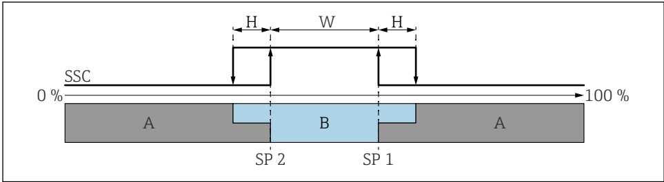
图 16 SSC, 双区间控制
