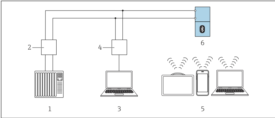
图 13 通过 IO-Link 进行远程操作
