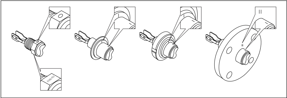
图 10 参照标记水平安装在罐体中的叉体位置
