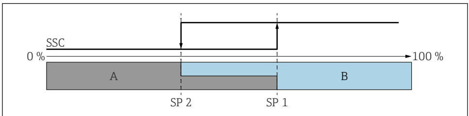
图 14 SSC，两点模式
