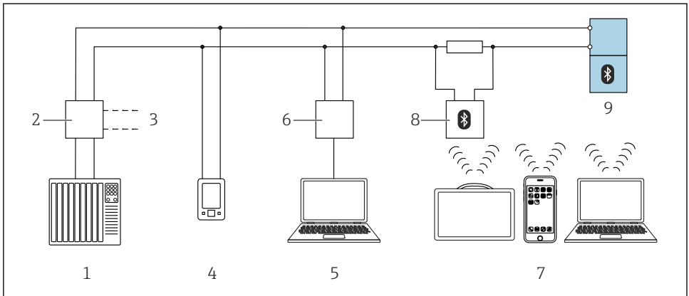
14 Options pour la configuration à distance via protocole HART
