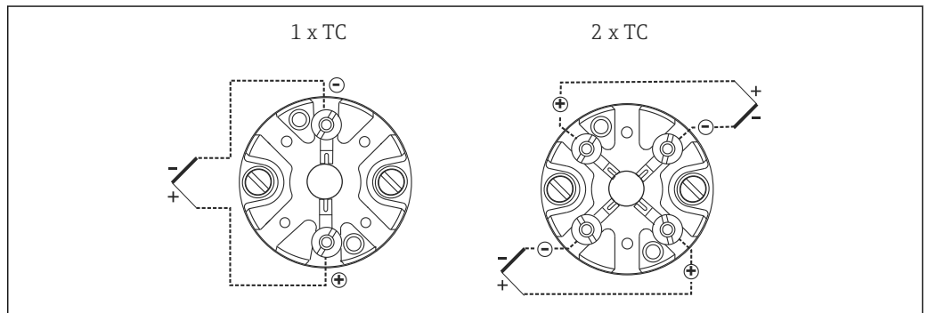
图 7 已安装陶瓷端子接线块
