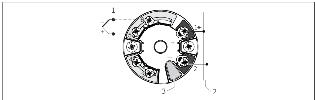
图 9 TMT7x 模块化温度变送器 (单输入通道)
