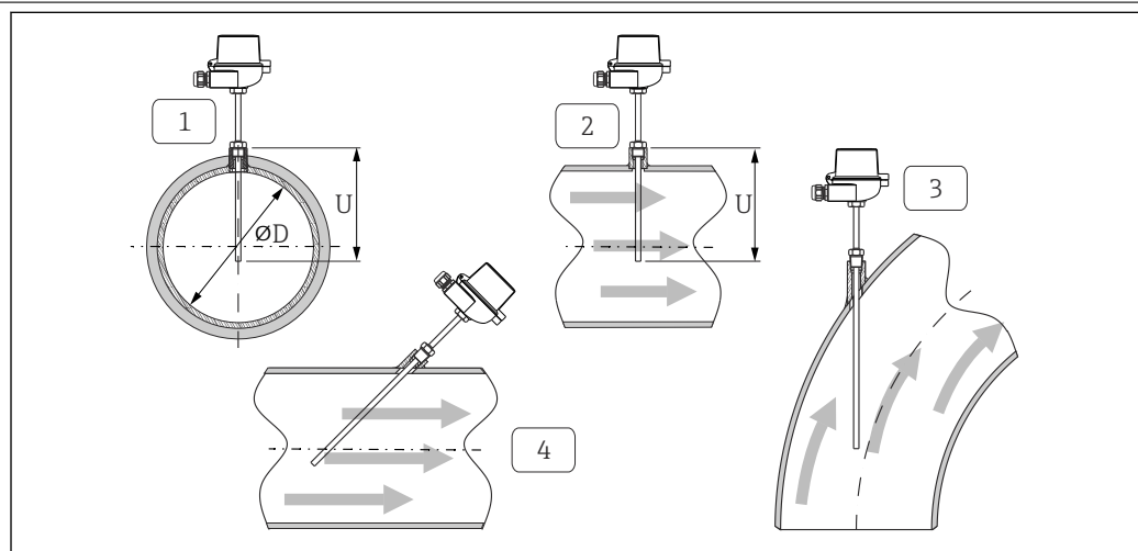
图 12 安装实例
