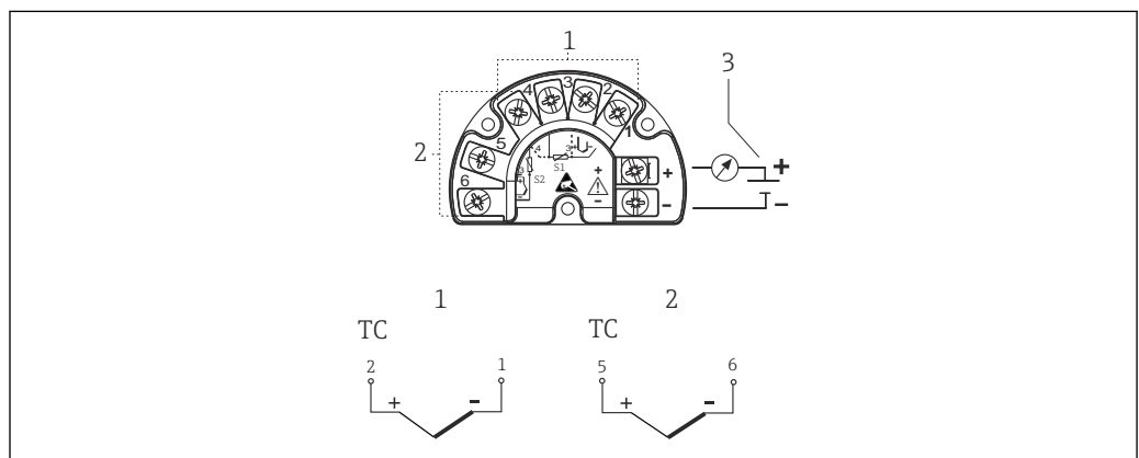
图 10 已安装 TMT162 或 TMT142B 现场型温度变送器
