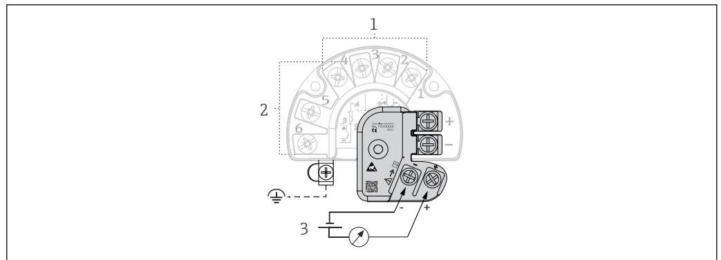
图 11 浪涌保护器的电气连接示意图
