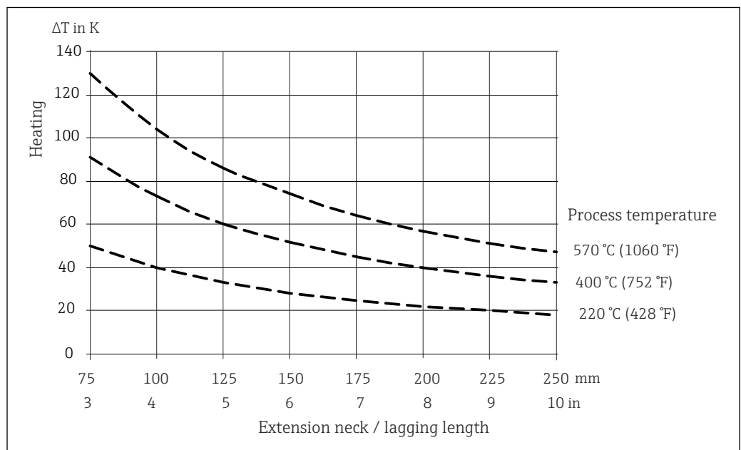
图 14 接线盒温度与过程温度的关系曲线。接线盒温度 = 环境温度 20 °C (68 °F) + \Delta T
