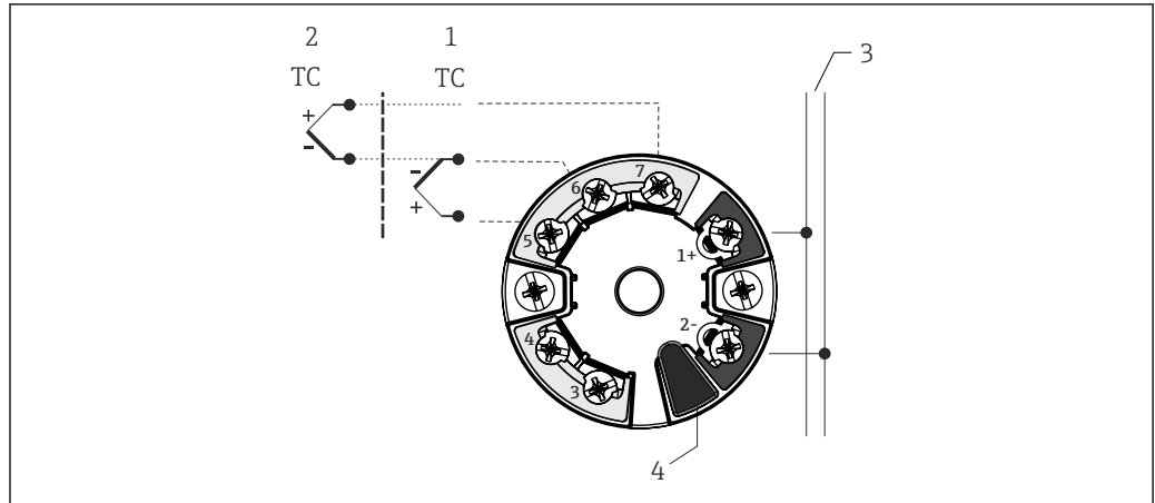
图 8 TMT8x 模块化温度变送器 (双路传感器输入)
