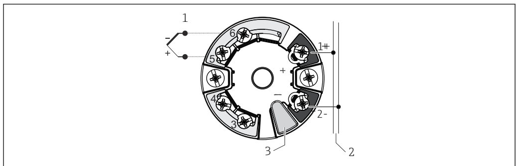
图 12 TMT7x 模块化温度变送器 (单输入通道)
