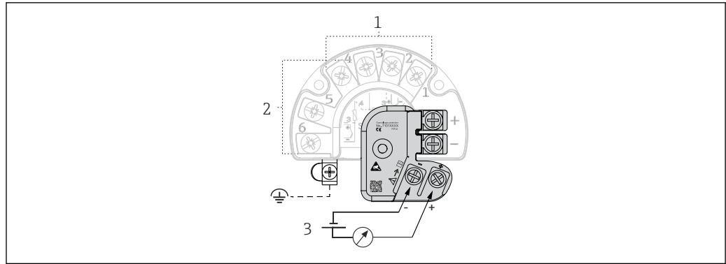
图 14 浪涌保护器的电气连接示意图
