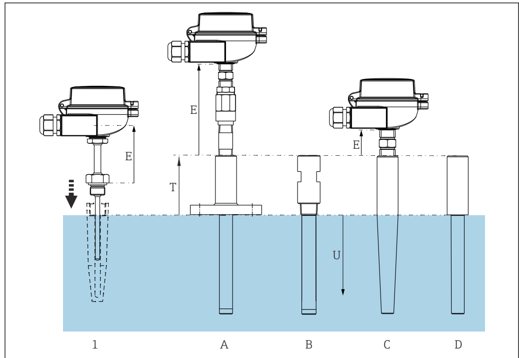
图 2 配置不同保护套管的温度计
