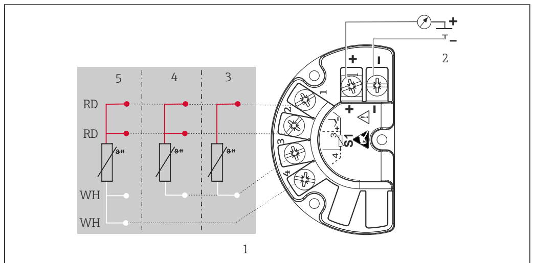
图 9 TMT142B (单输入通道)
