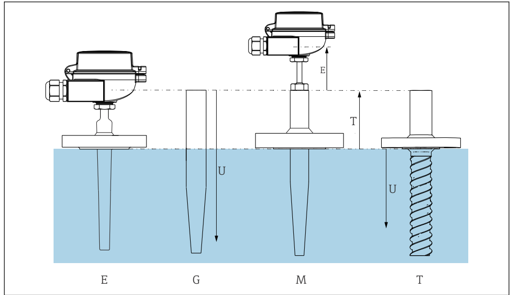
图 3 配置不同保护套管的温度计
