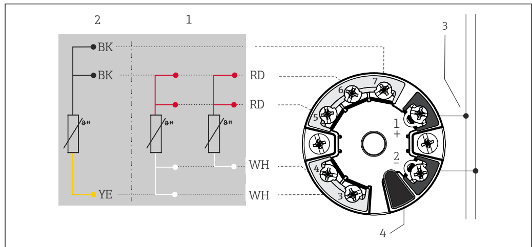
图 7 TMT8x 模块化温度变送器 (双路传感器输入)
