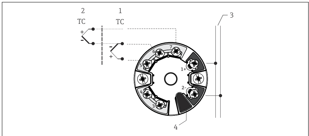
图 11 TMT8x 模块化温度变送器 (双路传感器输入)
