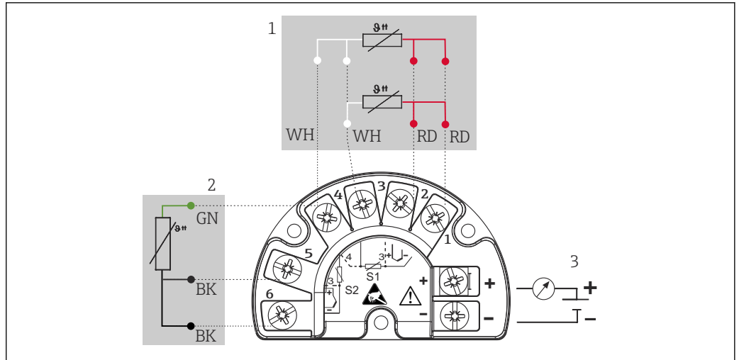
图 8 TMT162 (双输入通道)
