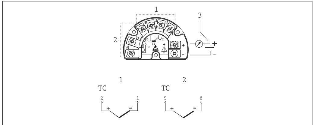
图 13 已安装 TMT162 或 TMT142B 现场型温度变送器
