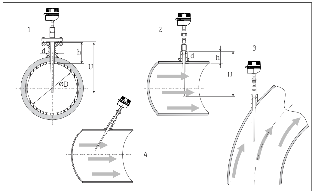
图 15 安装实例
