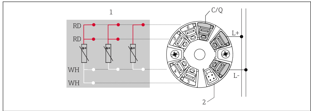
图 6 TMT36 模块化温度变送器 (单输入通道)
