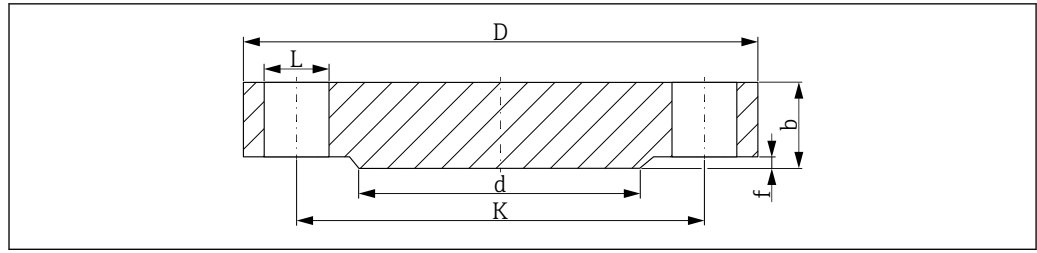
图 21 密封面形式: RF 突面 (B1 型)
