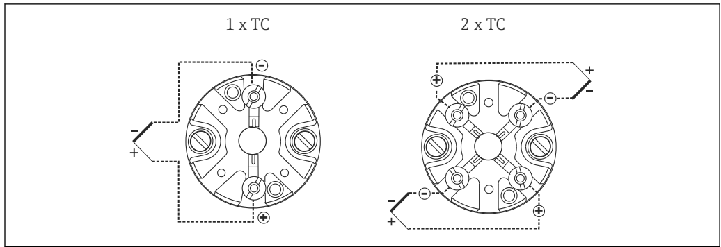
图 10 已安装陶瓷端子接线块
