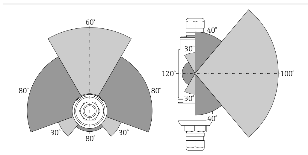
図 3 伝送窓の位置による範囲の違い
