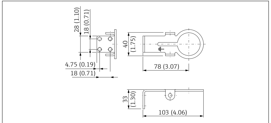
図 19 固定ブラケットの寸法 - 壁面取付け
