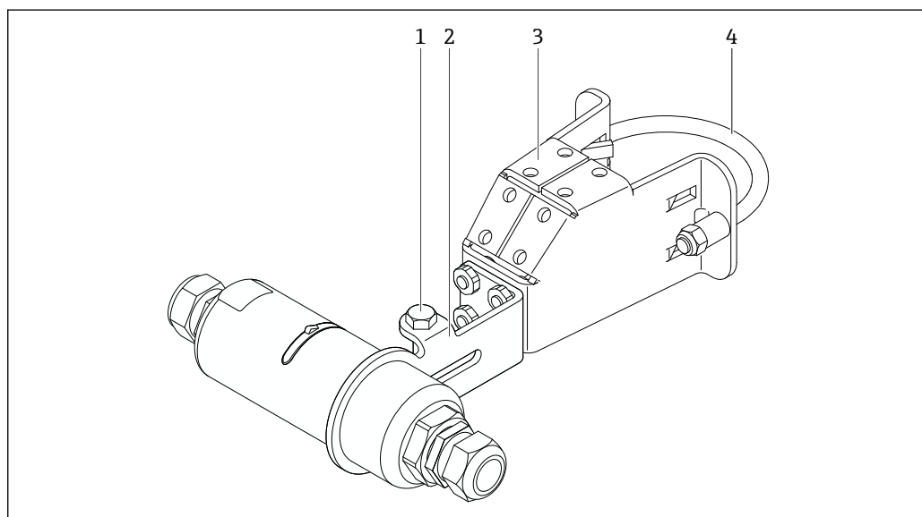
図 16 取付金具（オプション）を使用した FieldPort SWA50 の取付け
