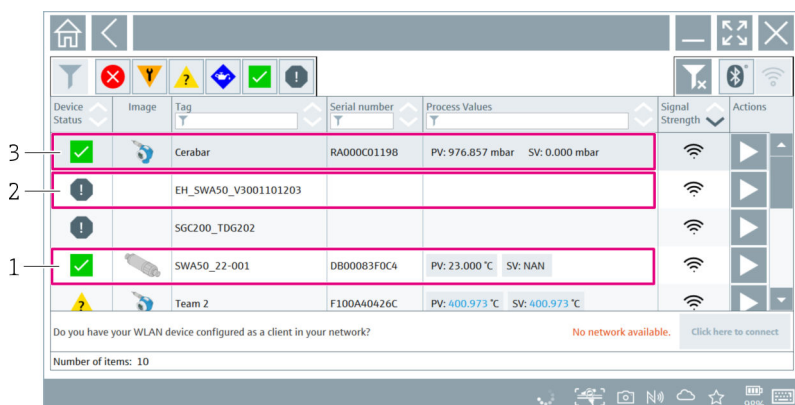
19 Appareils accessibles (liste des appareils joignables)
