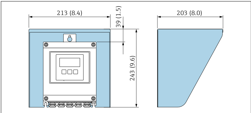
図 1 日除けカバー、寸法：mm (in)
