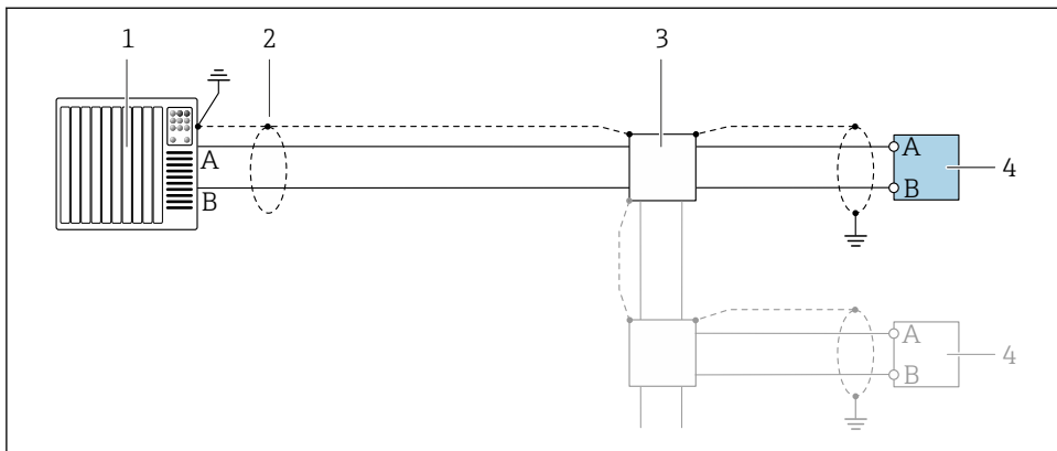
図 3 Modbus RS485（非危険場所およびゾーン 2/Div. 2 用）の接続例
