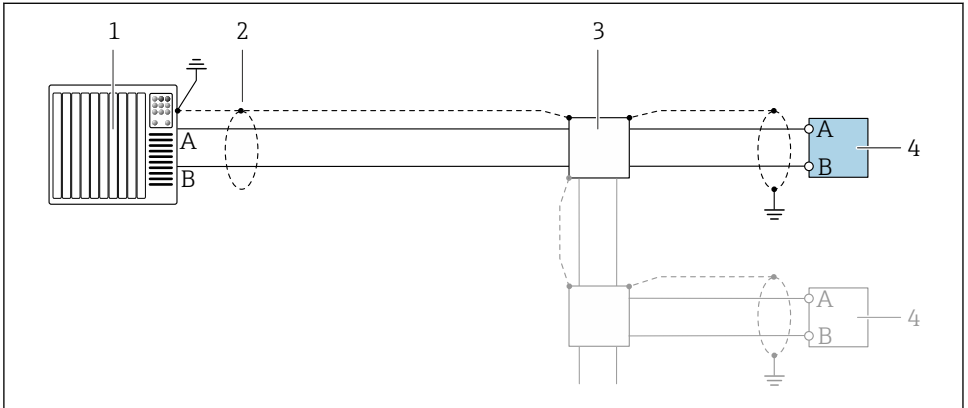
图 3 接线示例：Modbus RS485，非危险区和防爆 2 区/ Div. 2 防爆场合
