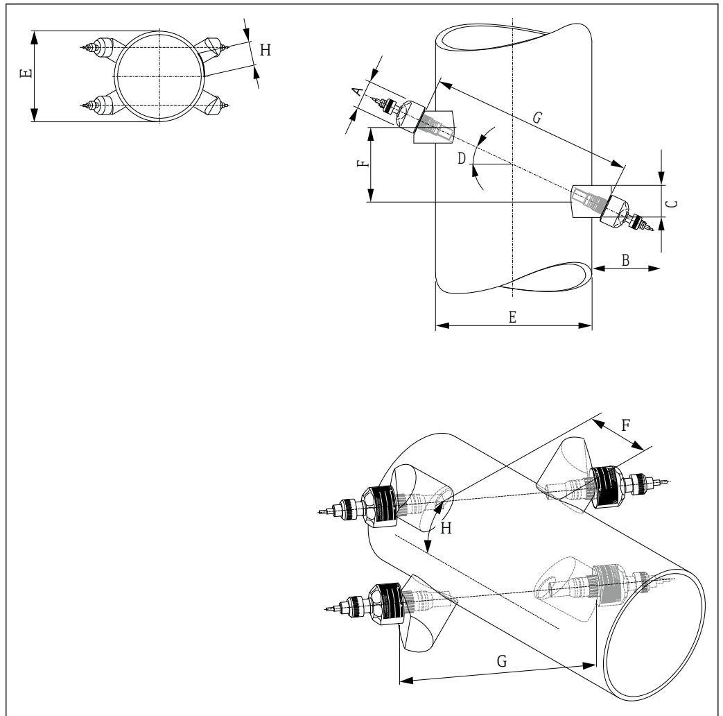
23 Versão de instalação de dois caminhos
