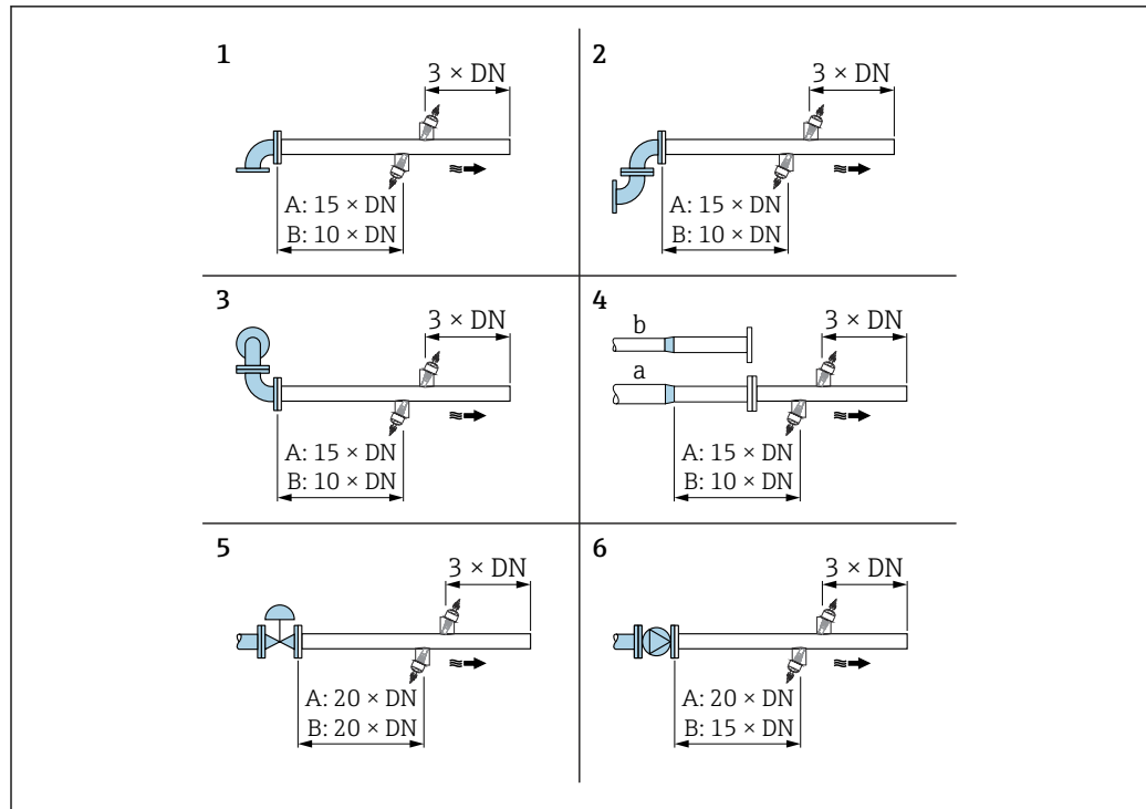
12 Trechos retos a montante e a jusante mínimos com diferentes obstruções na vazão (A: medição de caminho único, B: medição de dois caminhos)
