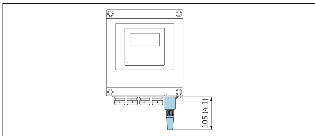
▣ 25 Unidade de engenharia mm (pol)
