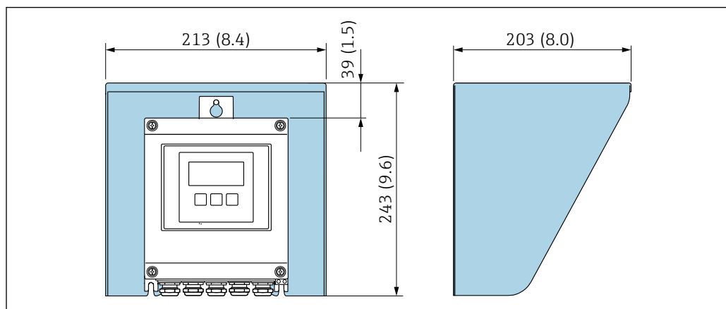
▣ 24 Tampa de proteção contra tempo; unidade de engenharia mm (pol.)
