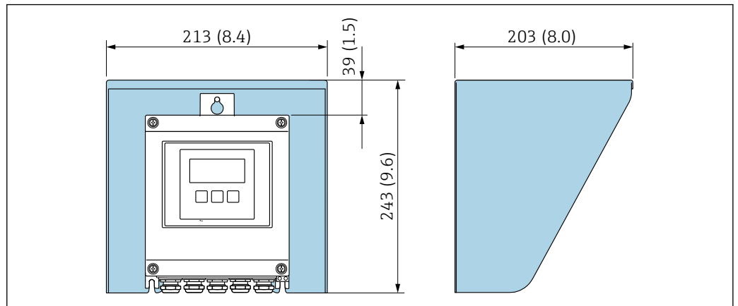
図 24 日除けカバー、寸法：mm (in)
