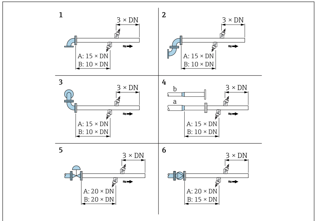
図 12 障害物が存在する場合の上流側/下流側の必要直管長 (A: 1 パス計測、B: 2 パス計測) (DN: 配管径)
