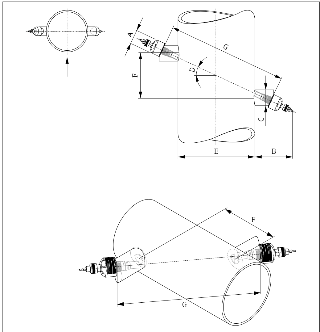
図 17 1 測線設置バージョン
