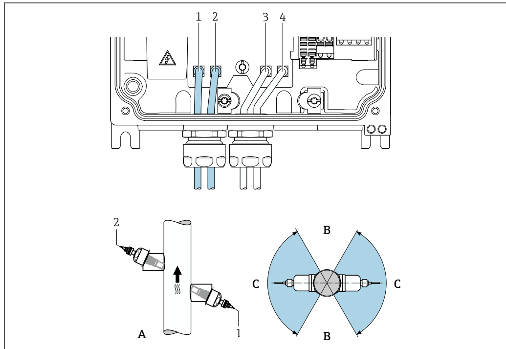
図 11 取付方向図
