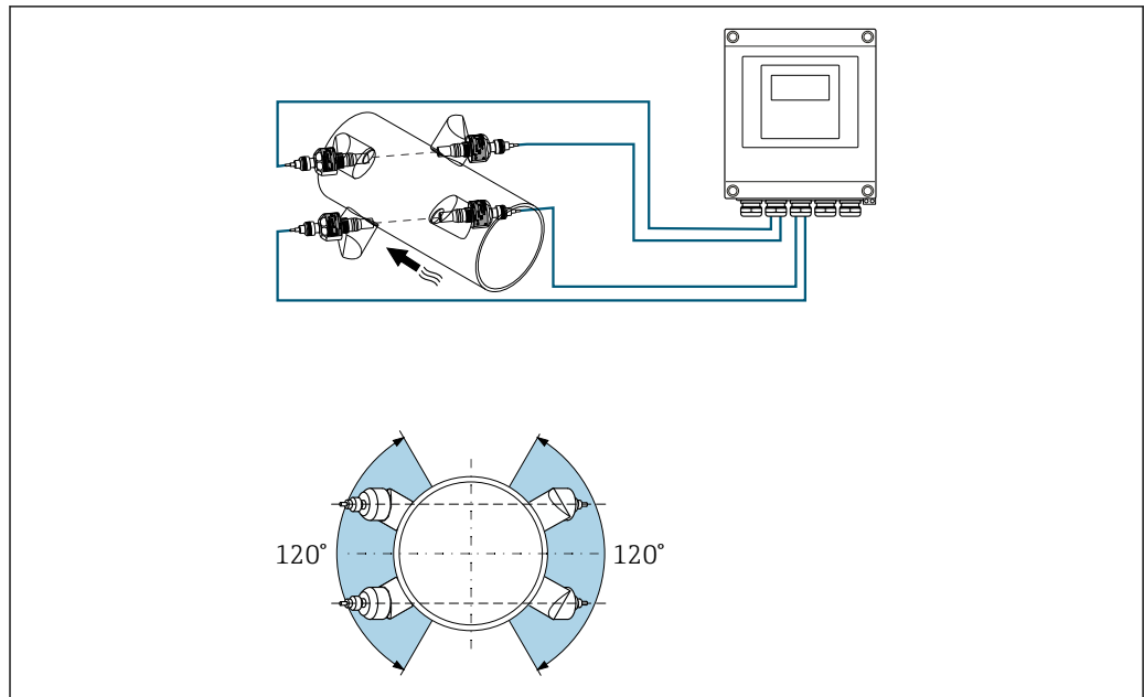
図 1 2パス計測：測定点におけるセンサセット水平配置の例
