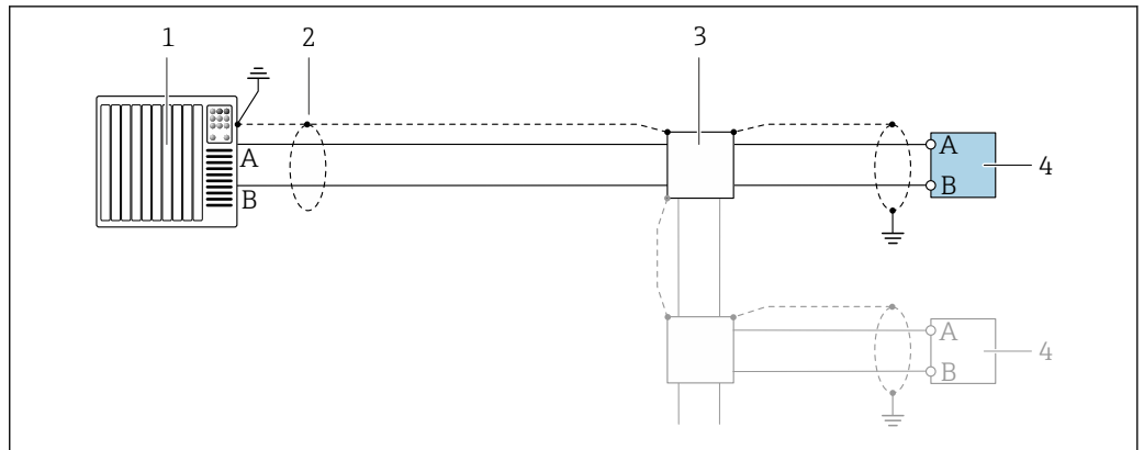
図 7 Modbus RS485（非危険場所およびゾーン 2/Div. 2 用）の接続例
