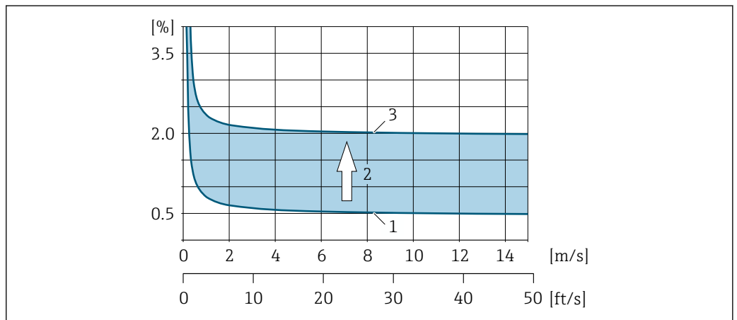
図 9 呼び口径 200A (8") 以上の配管における測定誤差の例
