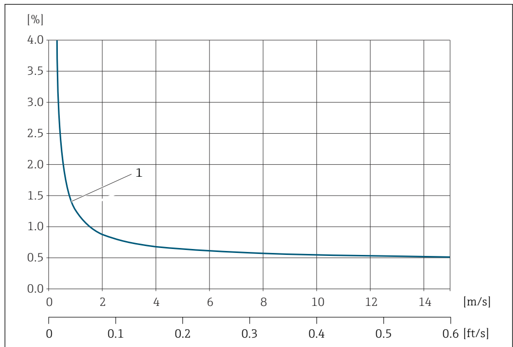
図 10 最大測定誤差の例 (体積流量) (% o.r.)
