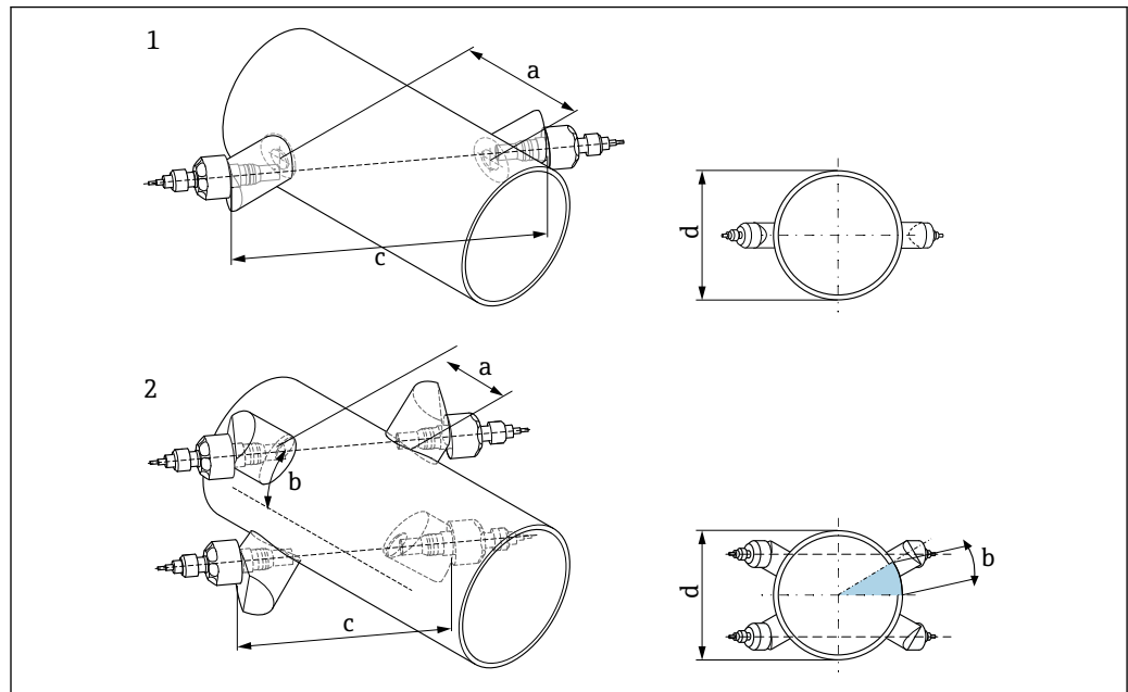
図 13 取付に関する用語の説明
