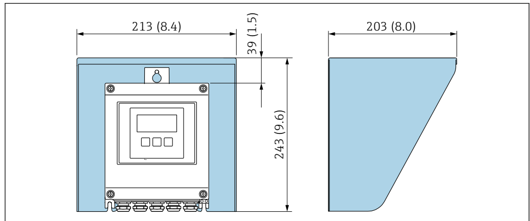
図 19 日除けカバー、寸法：mm (in)
