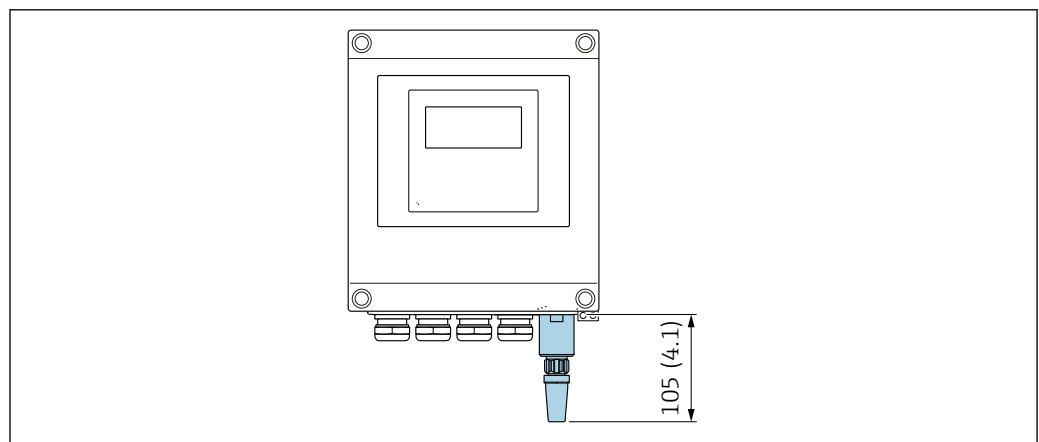
図 20 単位 mm (in)
