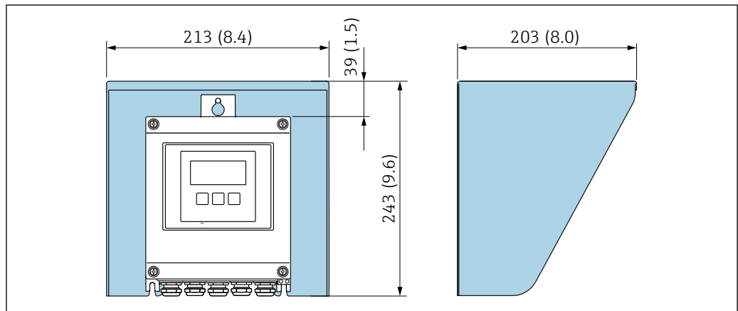
図 16 日除けカバー、寸法 : mm (in)
