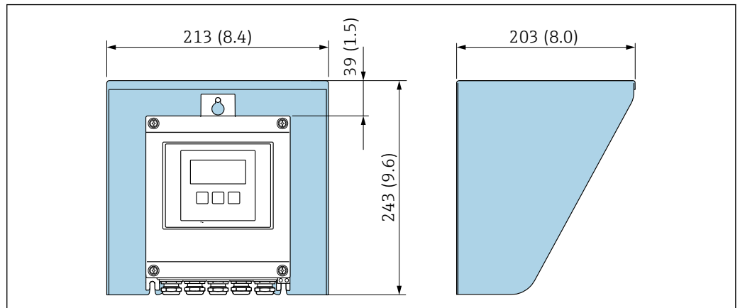
图 24 防护罩的外形尺寸示意图；单位：mm (in)
