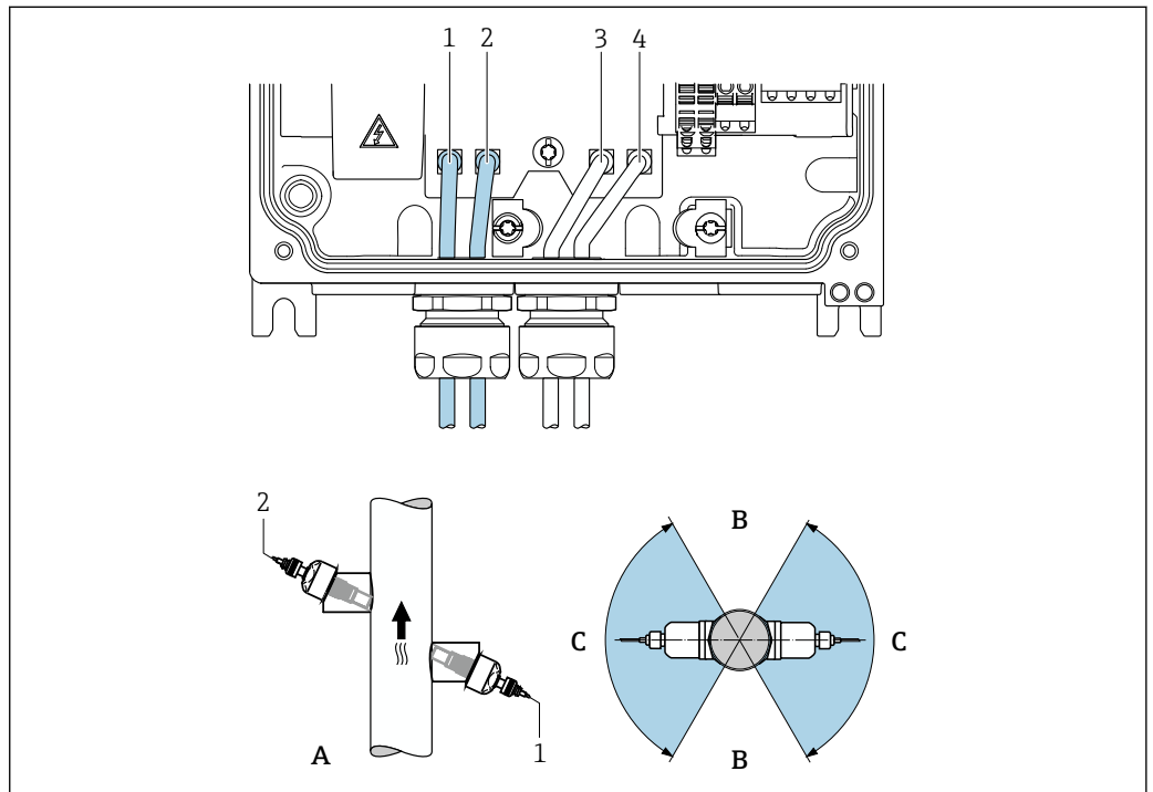
图 11 安装方向视图
