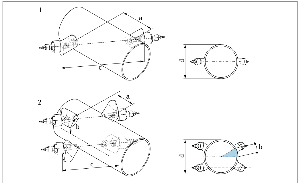
图 13 安装术语说明
