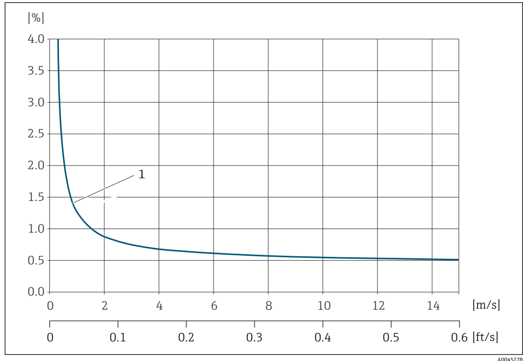
图 10 最大测量误差（体积流量）(% o.r.)的计算实例
