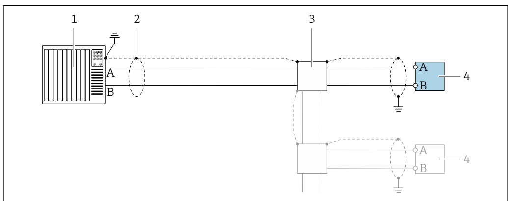
图 7 接线示例：Modbus RS485，非危险区和防爆 2 区 / Div. 2 防爆场合
