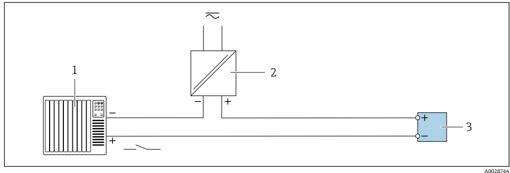
图 17 接线实例：状态输入
