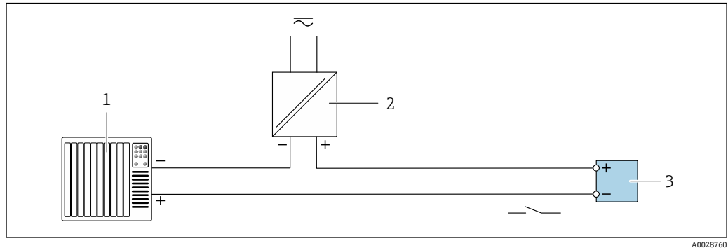
图 16 接线实例：开关量输出（无源信号）
