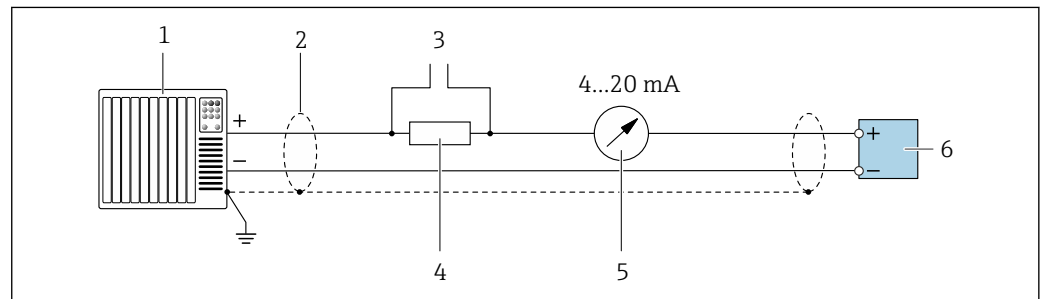
图 14 4...20 mA HART 电流输出 (有源) 的接线图
