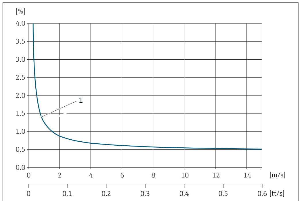
图 31 最大测量误差 (体积流量) (% o.r.) 的计算实例
