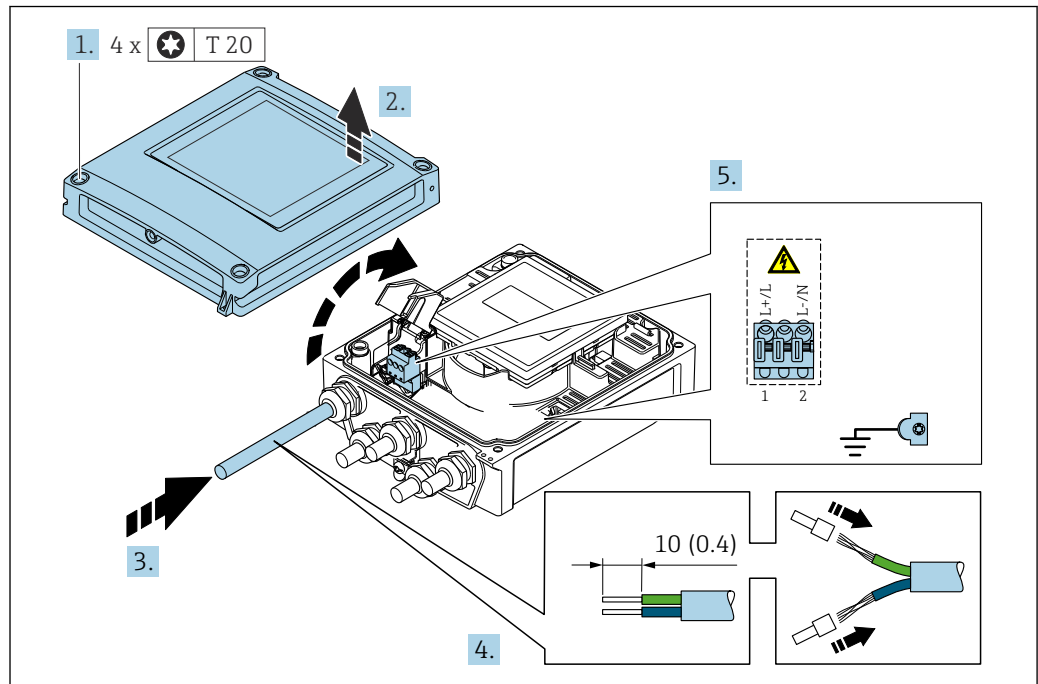
图 13 连接电源和带附加输出和输入的 0...20 mA / 4...20 mA HART
