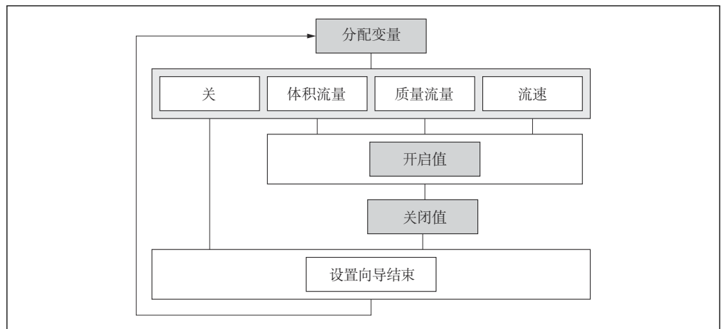
图 25 “设置”菜单中的“小流量切除”设置向导
