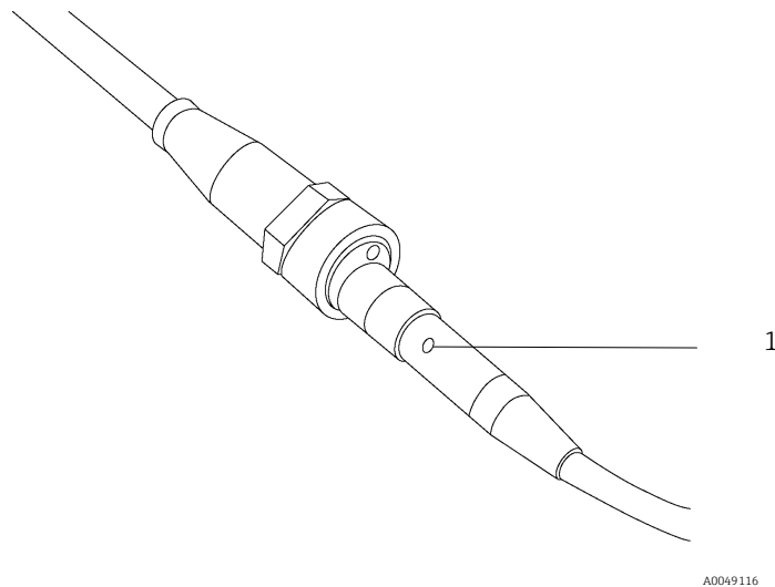
Figure 2. Indicateur d'émission laser sur la coque de raccordement de la fibre en acier inoxydable intégrée (1)
