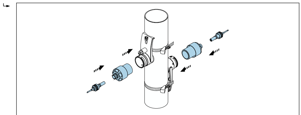
图 37 安装传感器并连接传感器电缆
