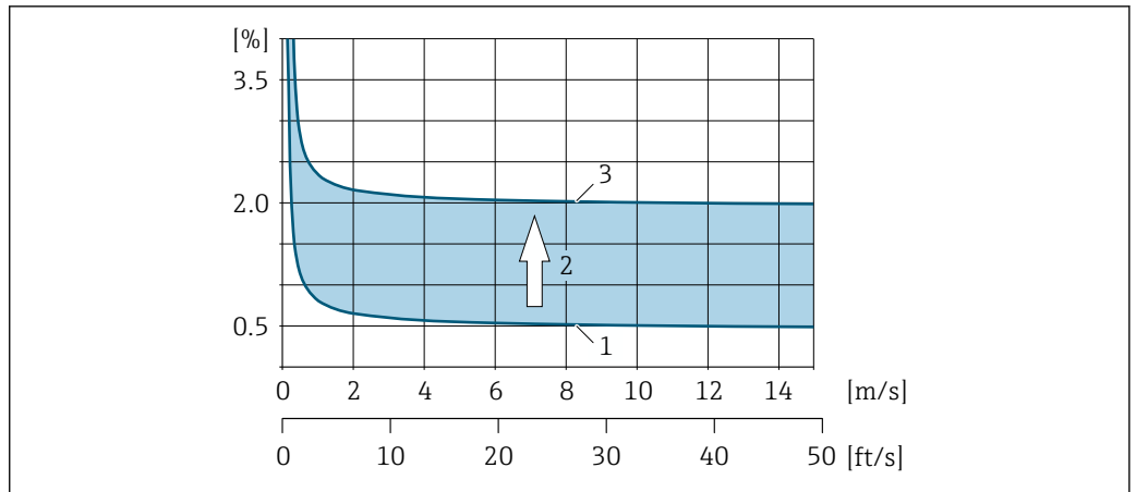
图 69 公称口径 DN > 200 (8")的管道中的绝对测量误差实例
