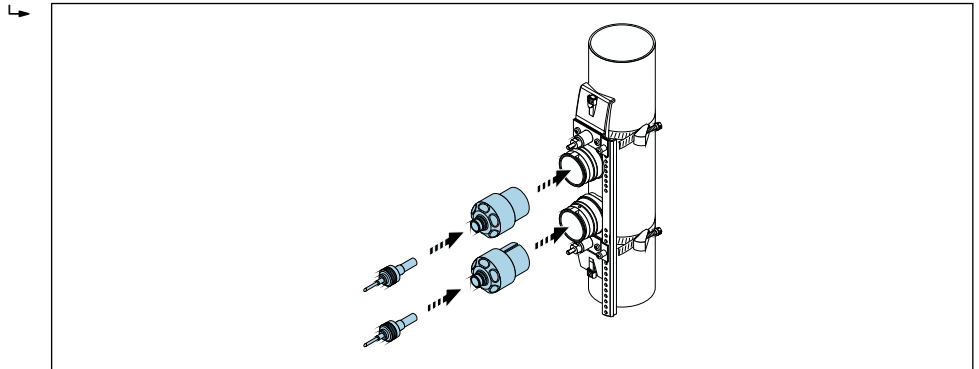
图 40 安装传感器并连接传感器电缆
