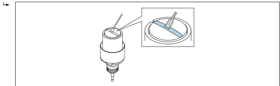
图 39 在传感器的接触面上涂抹耦合凝胶（如果没有耦合垫）
