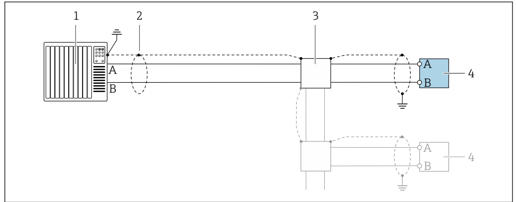
图 46 接线实例：Modbus RS485，非危险区和防爆 2 区；CI. I, Div. 2 防爆场合
