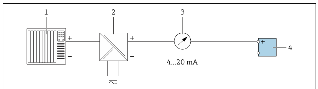
图 48 接线实例：4...20 mA 电流输出（无源信号）
