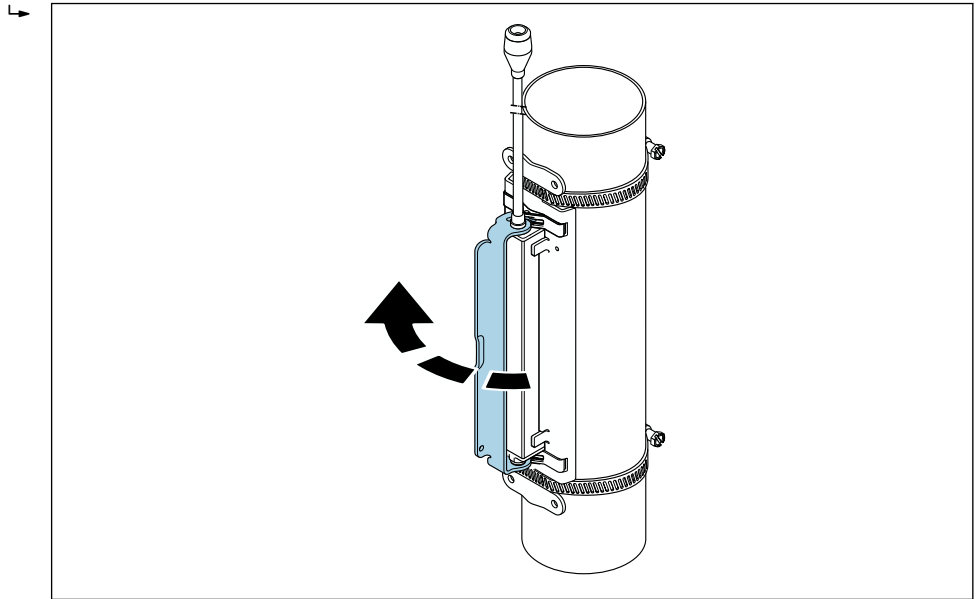
31 紧固传感器外壳
