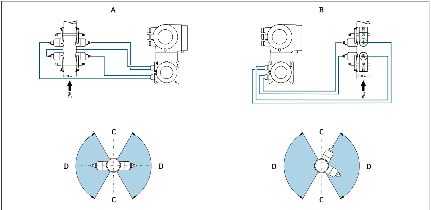
图 8 双声路测量：在测量点处水平布置传感器组的示意图
