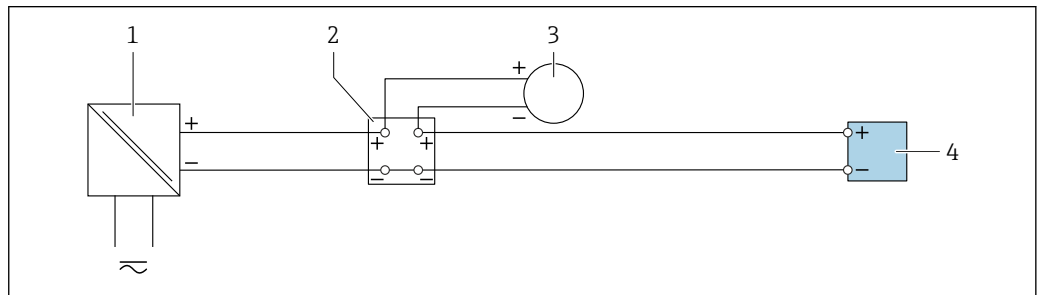
图 54 接线实例：4...20 mA 电流输入
