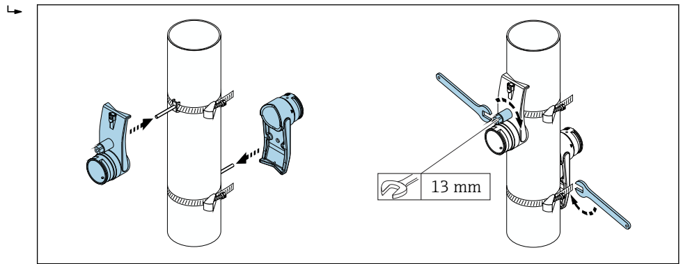
图 35 安装传感器安装支座
