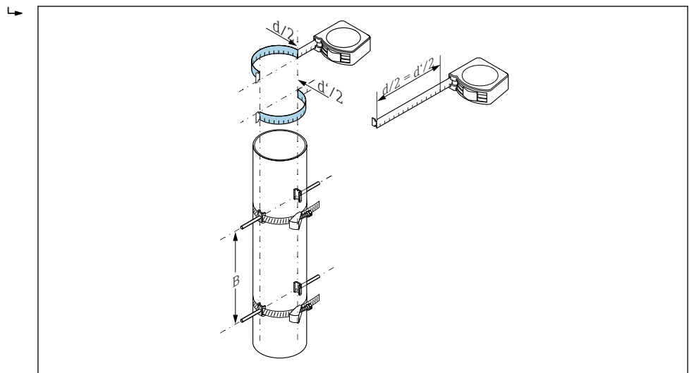
图 34 使用卷尺定位捆扎带和安装螺栓 (步骤 2...4)
