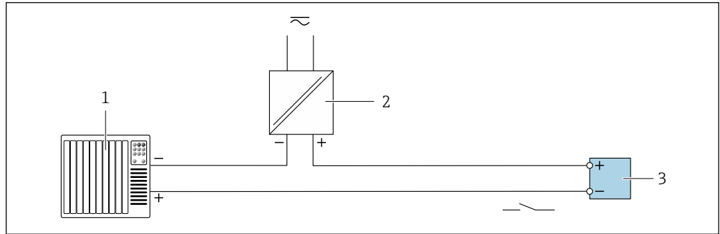
图 50 接线实例：开关量输出（无源信号）
