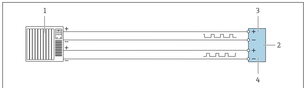
图 51 接线实例：脉冲（相移）输出（有源信号）
