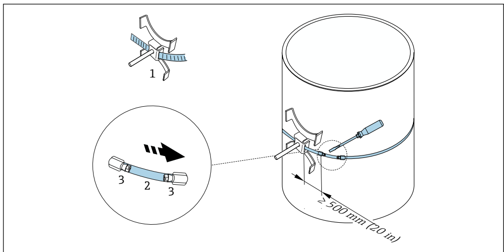
图 27 带捆扎带的传感器安装支座 (大公称口径)
