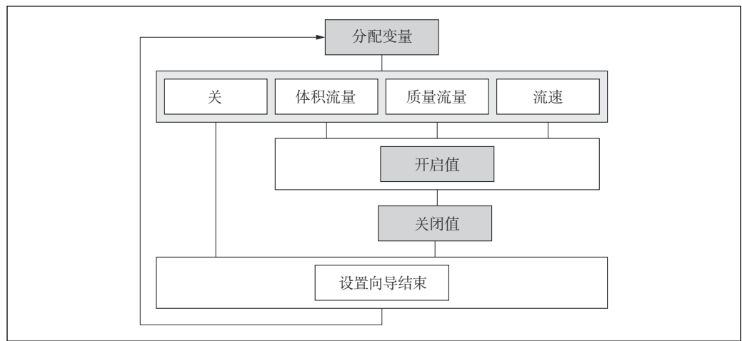
图 65 “设置”菜单中的“小流量切除”设置向导
