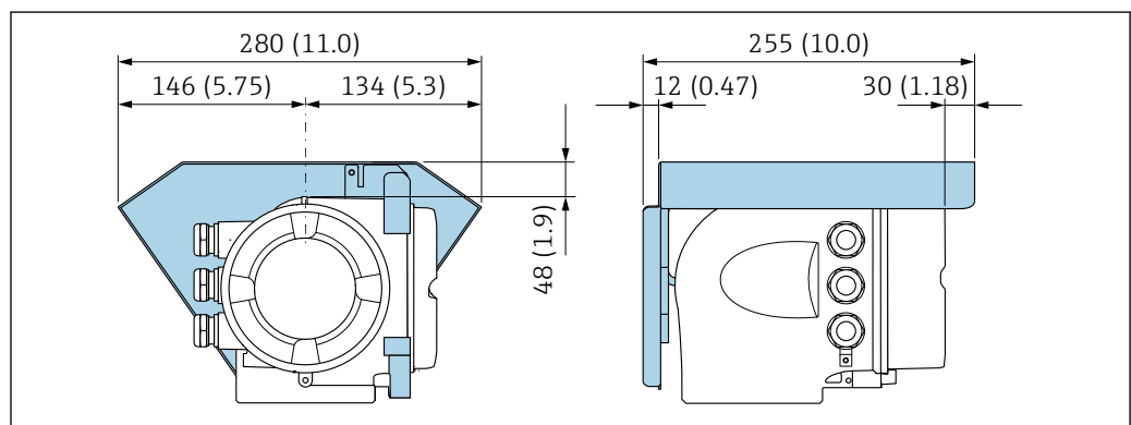
图 21 Proline 500 变送器的防护罩的外形尺寸图；单位：mm (in)
