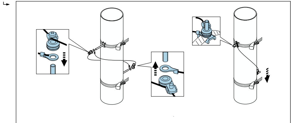
图 33 定位捆扎带 (步骤 2...4)
