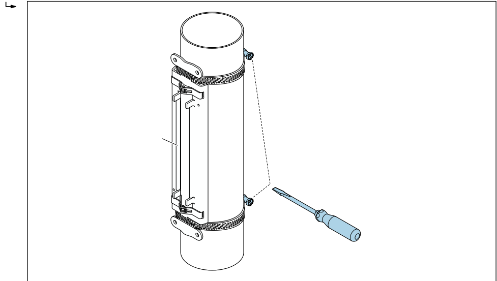
图 24 拧紧捆扎带的紧固螺丝。
