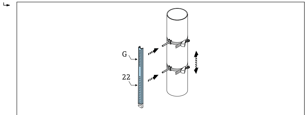
图 38 根据安装导轨确定距离（例如 G22）。
