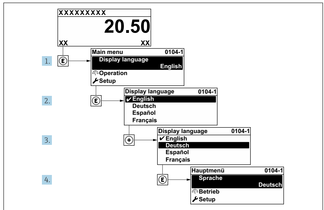
图 62 现场显示示意图
