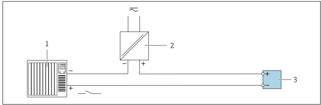
图 55 接线实例：状态输入
