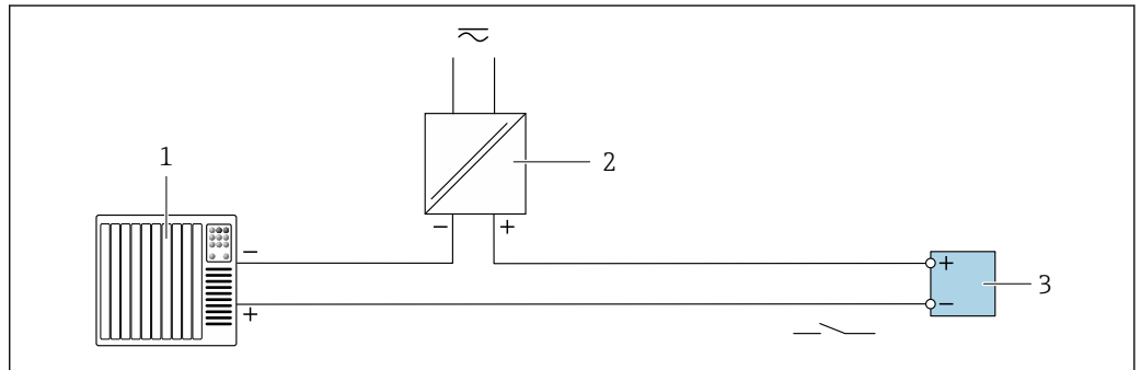
图 53 接线实例：继电器输出（无源信号）
