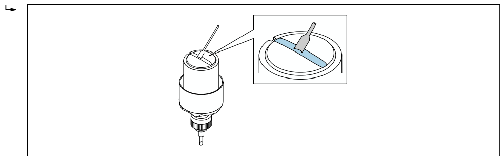
图 36 在传感器的接触面上涂抹耦合凝胶（如果没有耦合垫）
