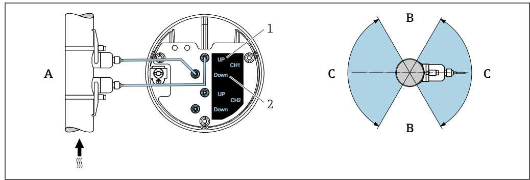
图 32 安装方向视图
