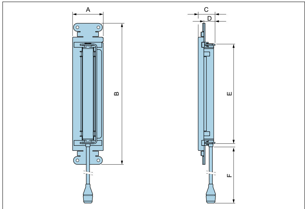
图 64 DN 1/2...2 1/2"
