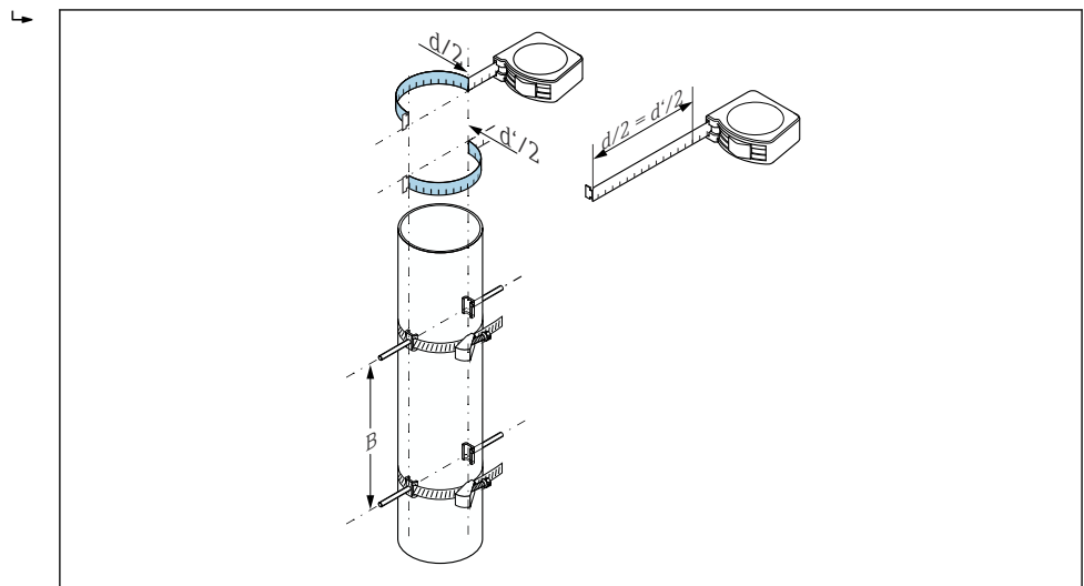
图 47 使用卷尺定位捆扎带和安装螺栓 (步骤 2...4)
