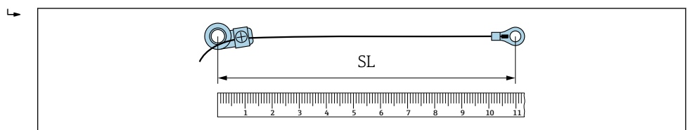
图 45 固定件与电缆接线头之间的距离等于测量线长度（SL）
