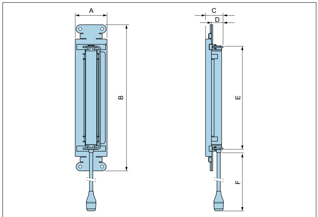
图 58 DN 15...65
