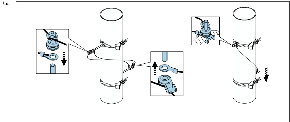
图 46 定位捆扎带 (步骤 2...4)
