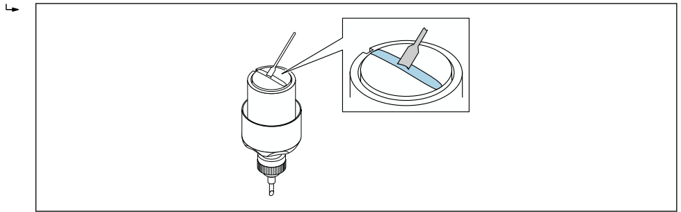
图 49 在传感器的接触面上涂抹耦合凝胶（如果没有耦合垫）
