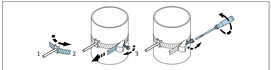
图 38 带捆扎带和铰接螺丝的传感器安装支座（中等公称口径）
