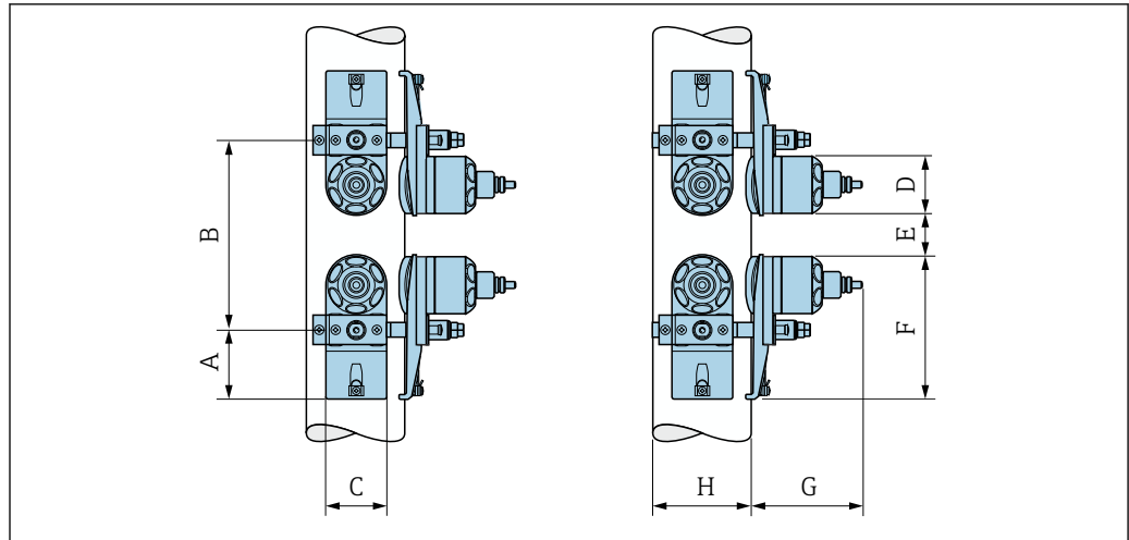
图 63 DN 2...160": 通过两组传感器测量
