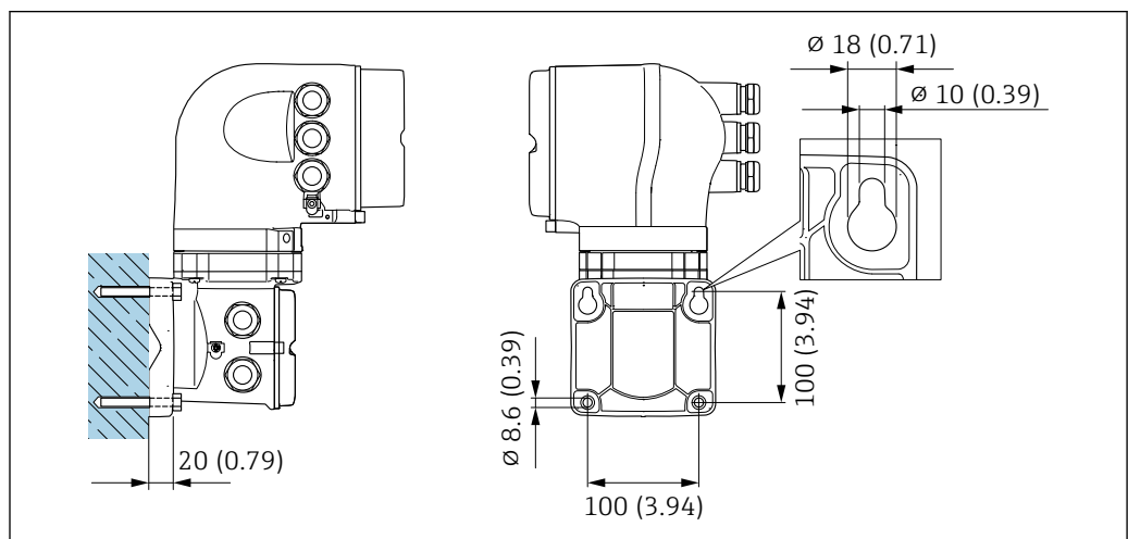
图 55 单位: mm (in)
