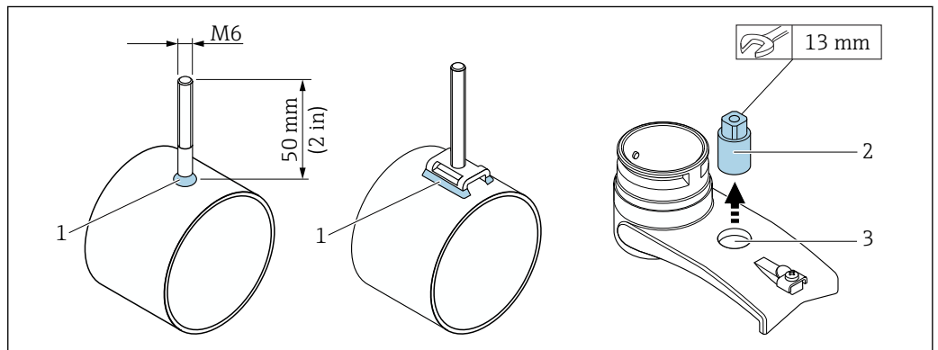
图 41 带焊接螺栓的传感器安装支座
