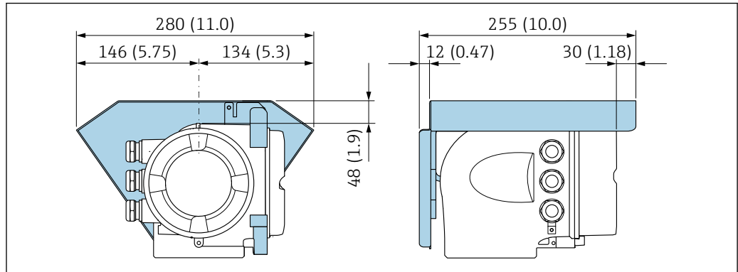
图 66 Proline 500 变送器的防护罩的外形尺寸图；单位：mm (in)
