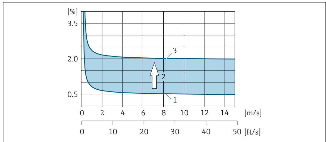
图 31 公称口径 DN > 200 (8") 的管道中的绝对测量误差实例
