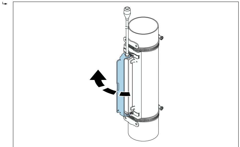
图 44 紧固传感器外壳
