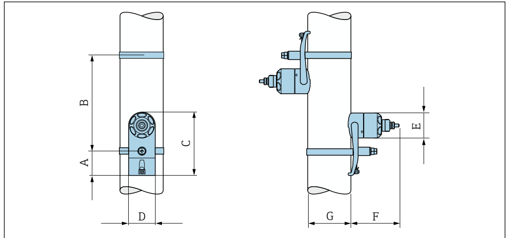
图 65 DN 2...160": 通过一组传感器测量
