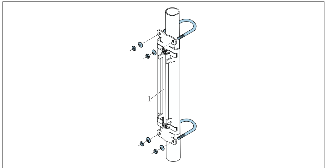
图 35 带 U 型螺丝的传感器安装支座
