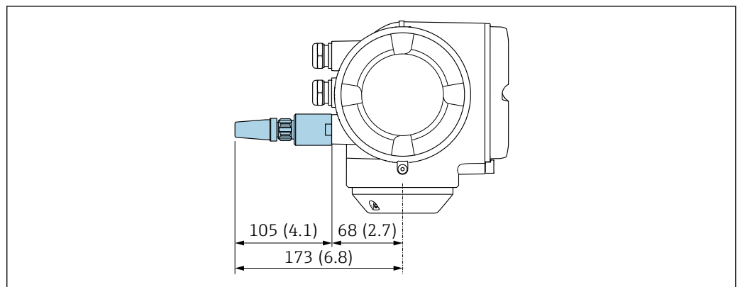
图 61 单位：mm (in)
