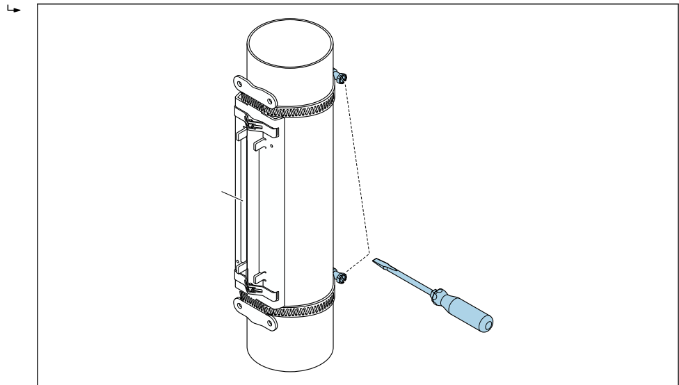
图 37 拧紧捆扎带的紧固螺丝。
