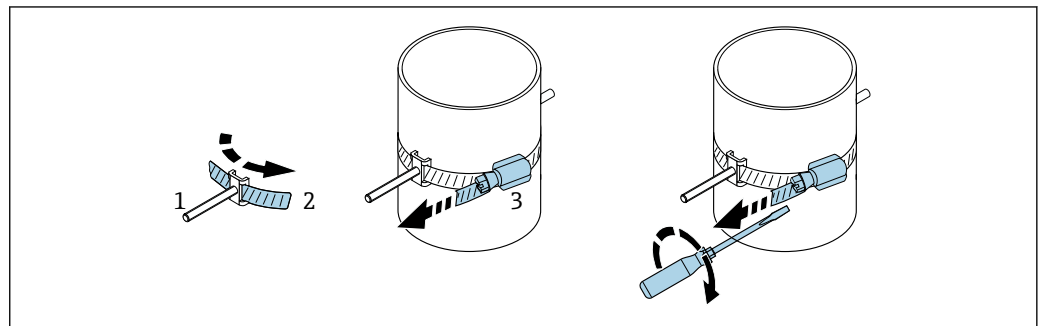
图 39 带捆扎带、不带铰接螺丝的传感器安装支座（中等公称口径）
