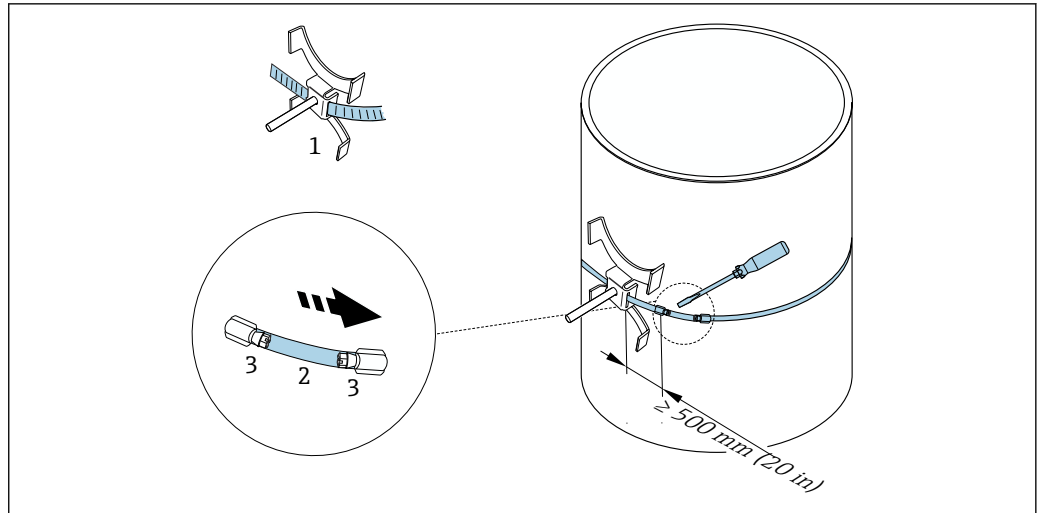
图 40 带捆扎带的传感器安装支座（大公称口径）
