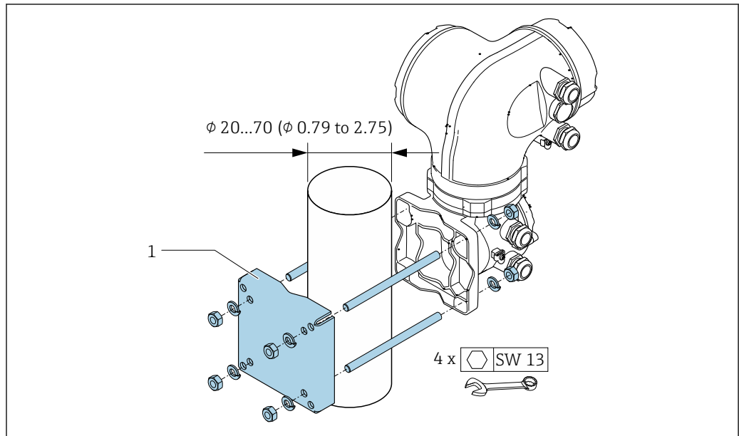
图 54 单位: mm (in)
