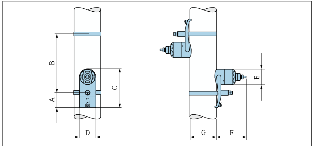
图 59 DN 50...4000: 通过一组传感器测量
