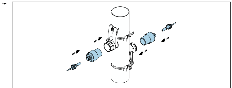
图 50 安装传感器并连接传感器电缆
