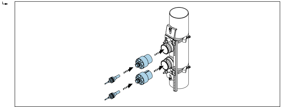
图 53 安装传感器并连接传感器电缆
