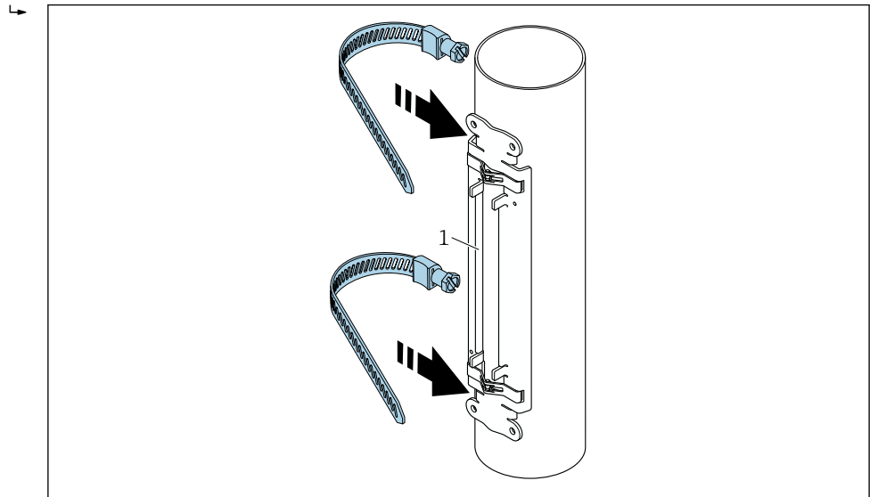
图 36 定位传感器安装支座并安装捆扎带。
