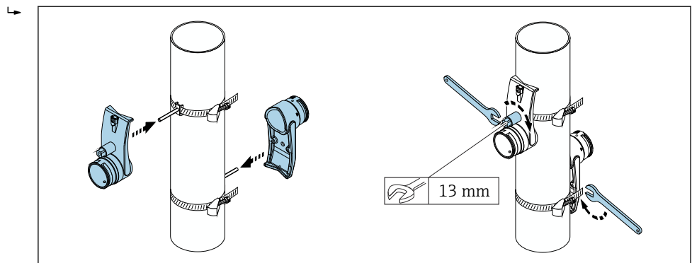
图 48 安装传感器安装支座
