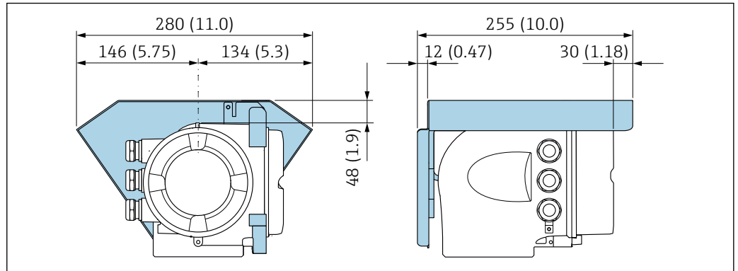
图 60 Proline 500 变送器的防护罩的外形尺寸图；单位：mm (in)
