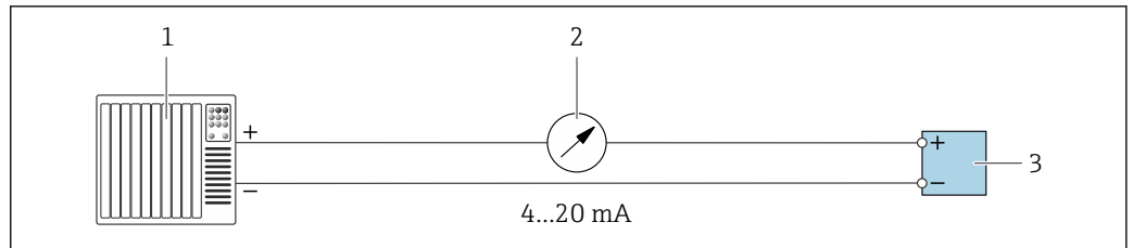
▣ 49 接线实例: 4...20 mA 电流输出 (有源信号)
