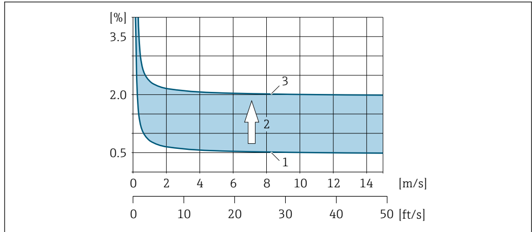
图 73 公称口径 DN > 200 (8") 的管道中的绝对测量误差实例
