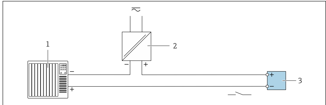
图 52 接线实例：开关量输出（无源信号）
