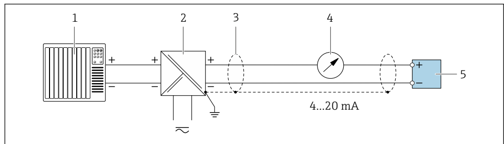
图 47 接线实例: 4...20 mA HART 电流输出 (无源信号)
