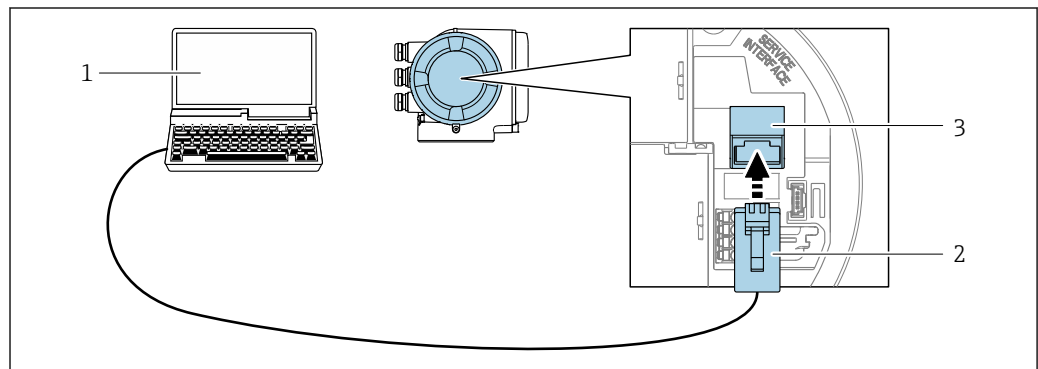
图 64 通过服务接口（CDI-RJ45）连接
