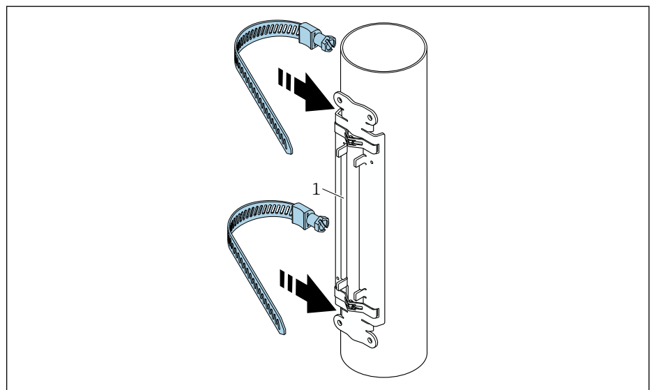
图 23 定位传感器安装支座并安装捆扎带。
