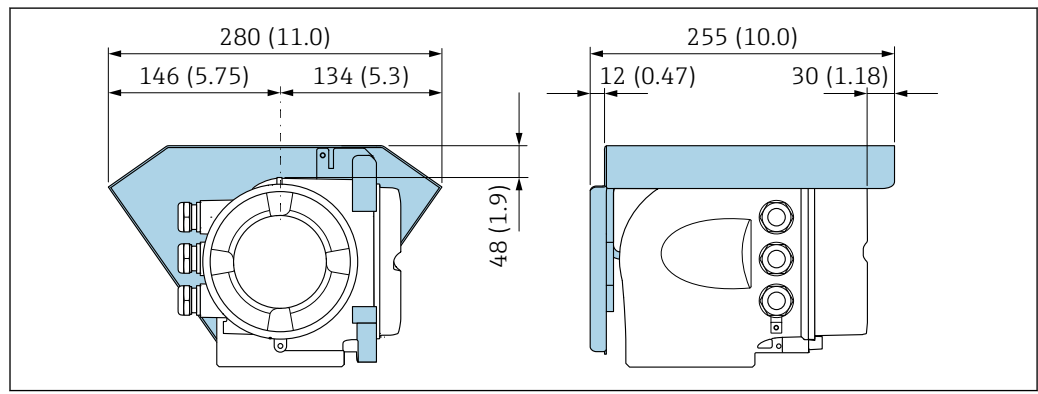
图 21 Proline 500 变送器的防护罩的外形尺寸图; 单位: mm (in)
