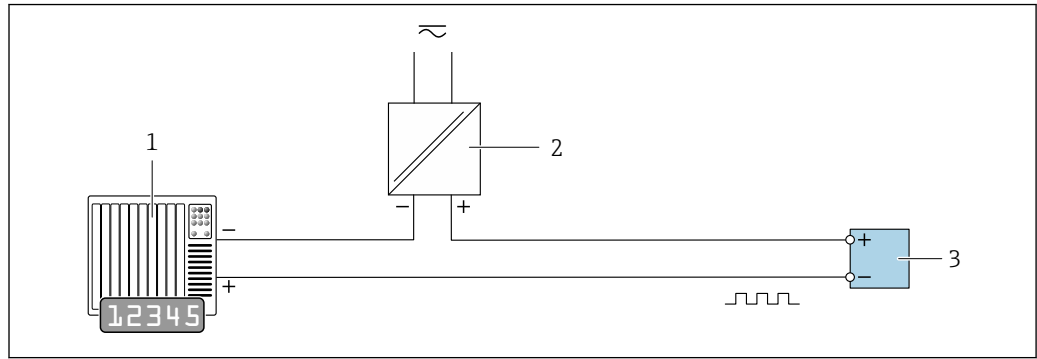
图 51 接线实例：脉冲/频率输出（无源信号）
