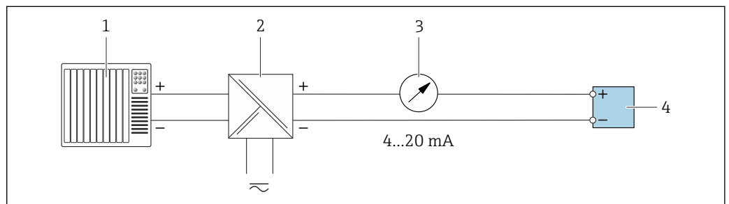
▣ 50 接线实例: 4...20 mA 电流输出 (无源信号)
