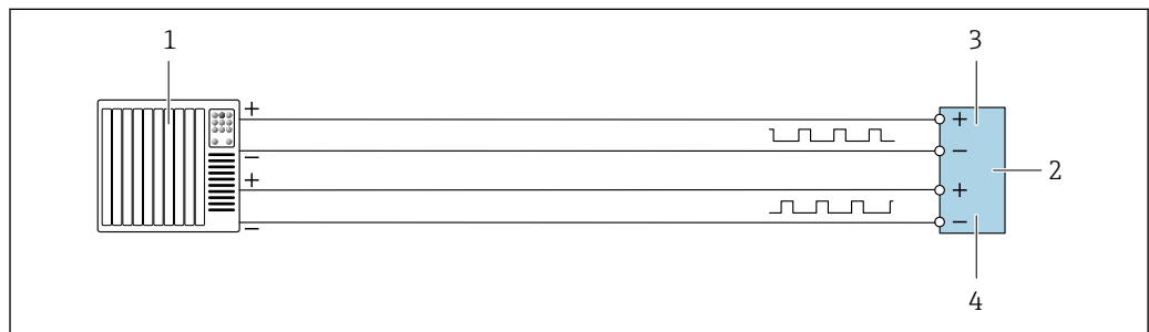
图 53 接线实例：脉冲（相移）输出（有源信号）
