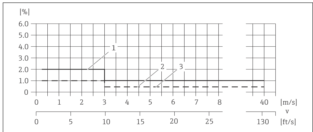
图 39 最大测量误差 (体积流量)，单位：读数百分比
