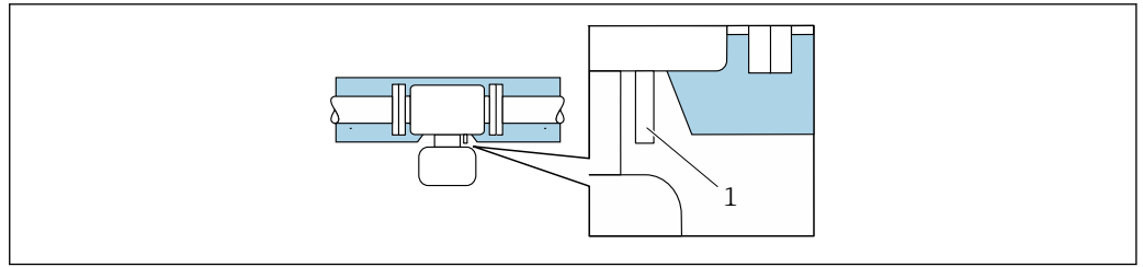
7 Isolation thermique avec tube prolongateur découvert et cellule de mesure de pression
