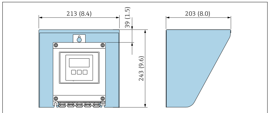
图 25 Proline 500 (数字) 变送器的防护罩的外形尺寸图; 单位: mm (in)
