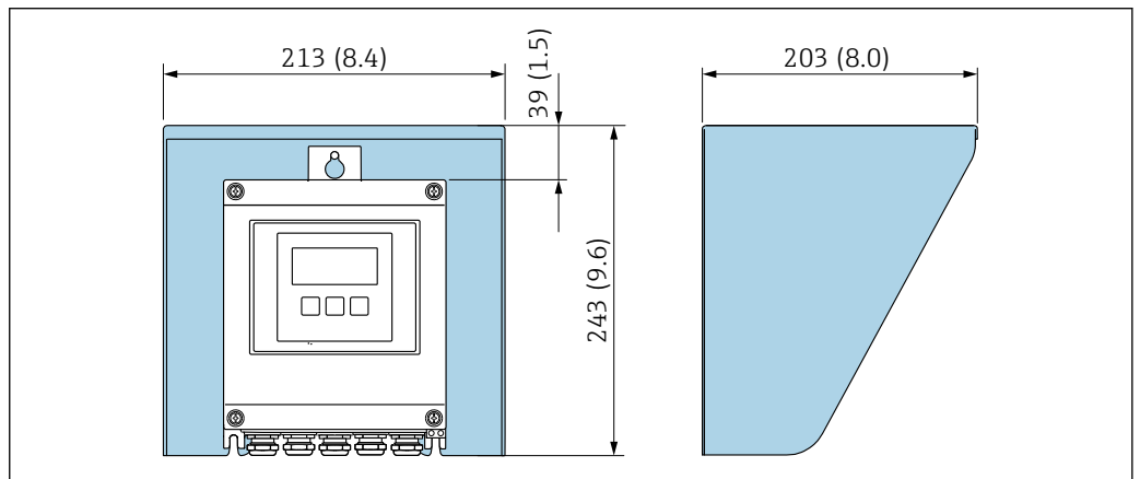
21 Proline 500 (数字) 变送器的防护罩的外形尺寸图; 单位: mm (in)
