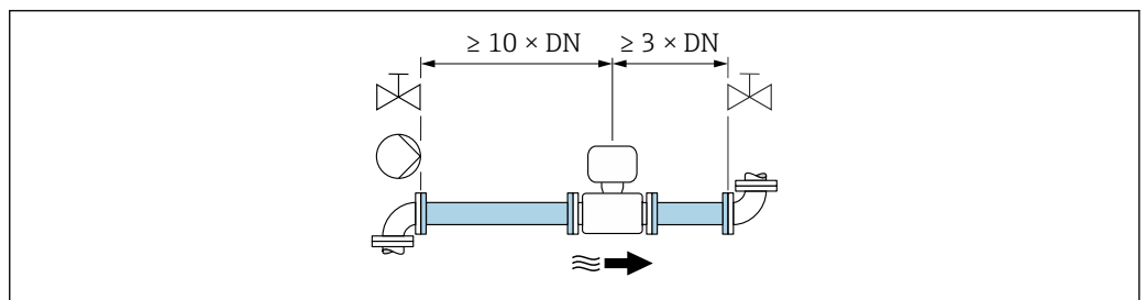
17 双声路型: 使用不同节流装置时的最小前后直管道长度。在订购选项“校准流量”中选择选型代号 A“1%”。
