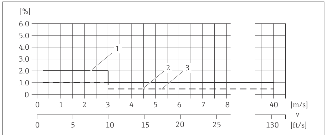
15 最大测量误差 (体积流量)，单位：读数百分比
