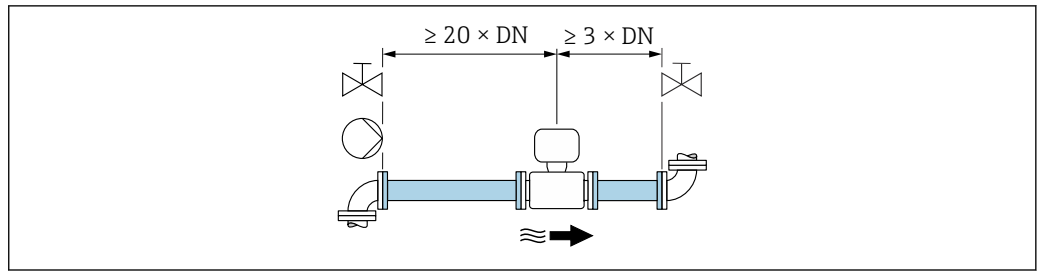
16 单声路型: 使用不同节流装置时的最小前后直管道长度。在订购选项“校准流量”中选择选型代号 A“1%”。
