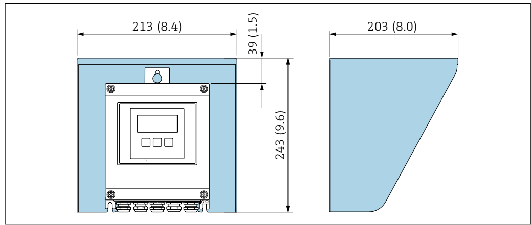
图 8 Proline 500 (数字) 变送器的防护罩的外形尺寸图; 单位: mm (in)
