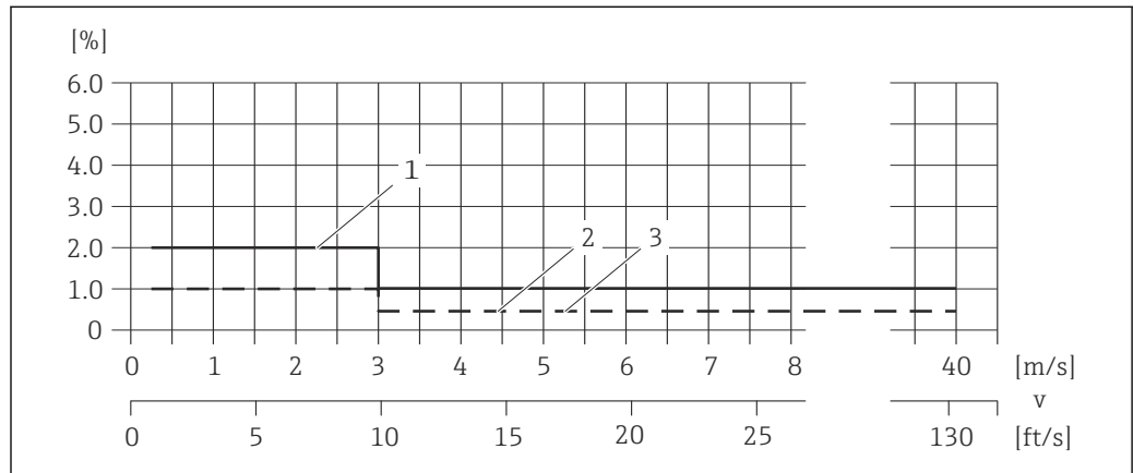
图 35 最大测量误差 (体积流量)，单位：读数值百分比
