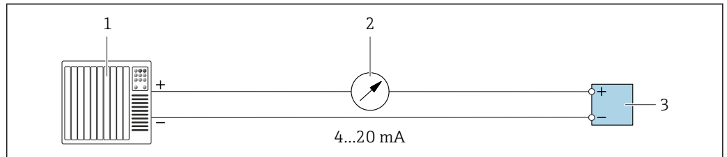
图 15 接线实例：4...20 mA 电流输出（有源信号）
