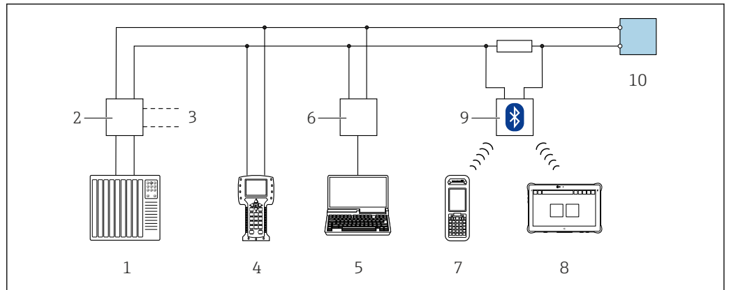
图 29 通过 HART 通信进行远程操作（无源信号）
