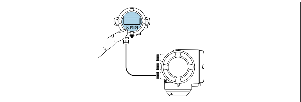
图 43 通过远传显示单元 DKX001 操作
