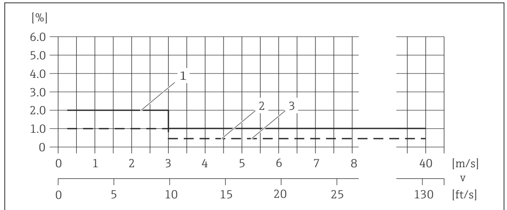
图 39 最大测量误差 (体积流量), 单位: 读数百分比
