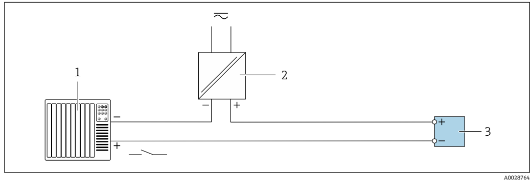
图 23 接线实例：状态输入
