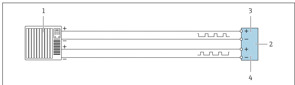
图 19 接线实例：双脉冲输出（有源信号）
