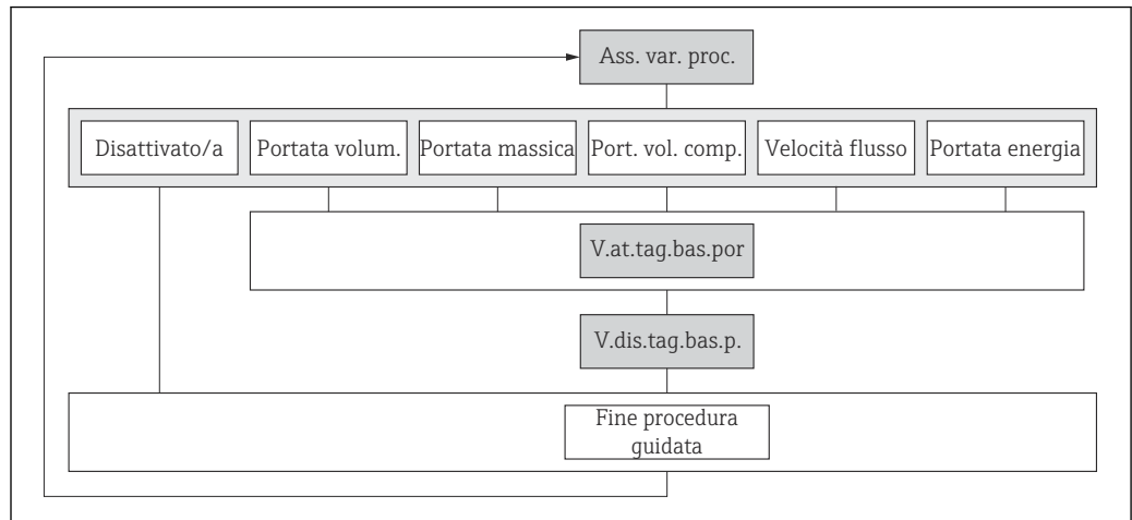
31 Procedura guidata "Taglio bassa portata" nel menu "Setup"
