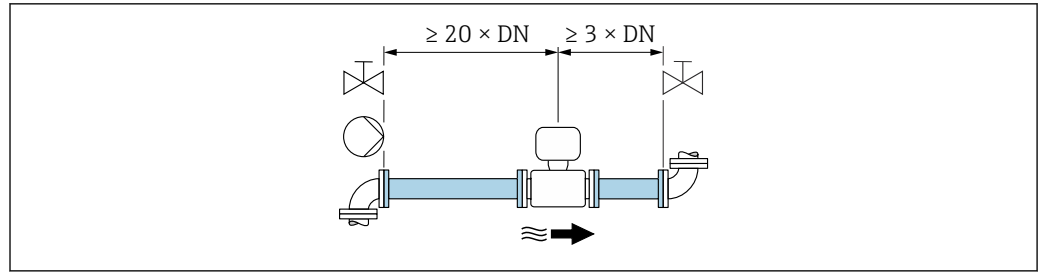
6 Versione a due vie: tratti rettilinei in entrata e in uscita minimi con vari elementi perturbatori Per codice d'ordine per "Taratura portata", opzione C "0.50%" e opzione D "0.50%", tracciabile secondo ISO/IEC17025".
